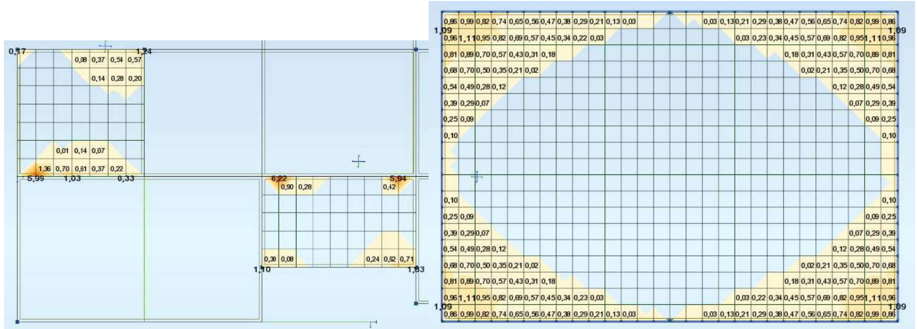
5.1.4 pav. Plokščių armavimas (Ay - viršutinis) (ašys 3-5, A) (ašys 3-5, A)
