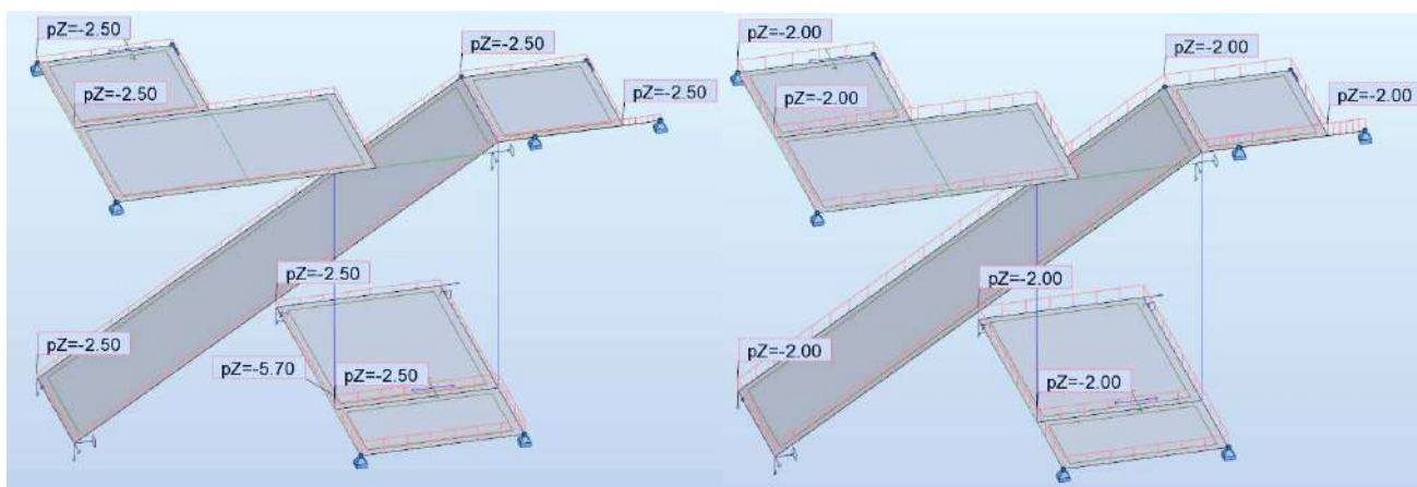
3.3.7 pav. Laiptinės ir perdangos apkrovų schema (DL2 ir LL1)
