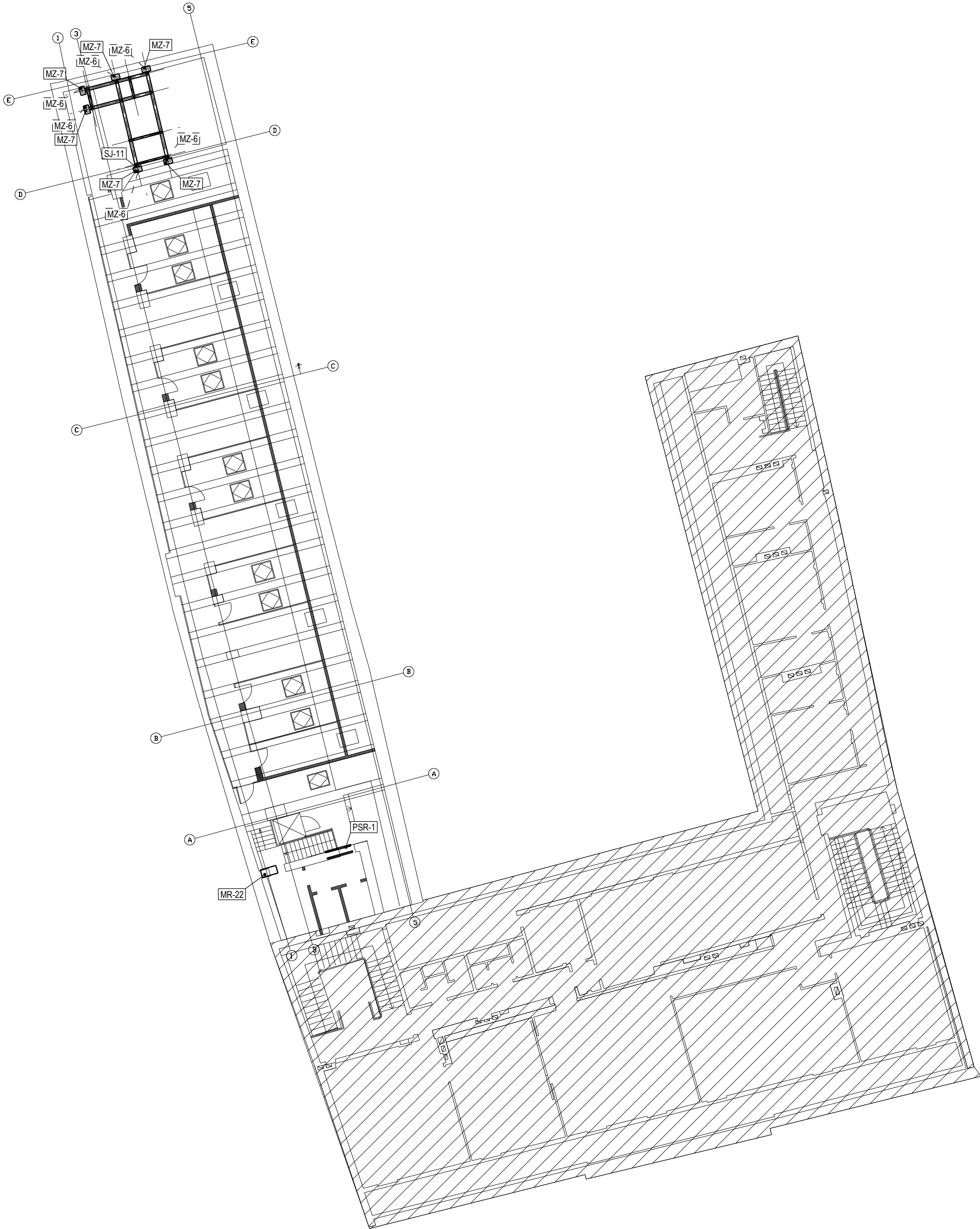
Pastato 4a. konstrukcijų planas M 1:200
