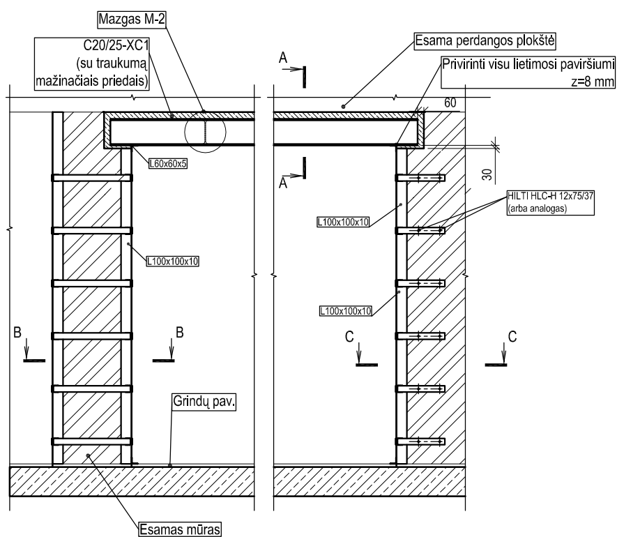
Principinis sijos įrengimas MDD-7 M1:50
