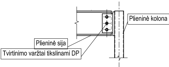
Principinis plieninių sijų sujungimo su plienine kolona mazgas M-4 M 1:20
