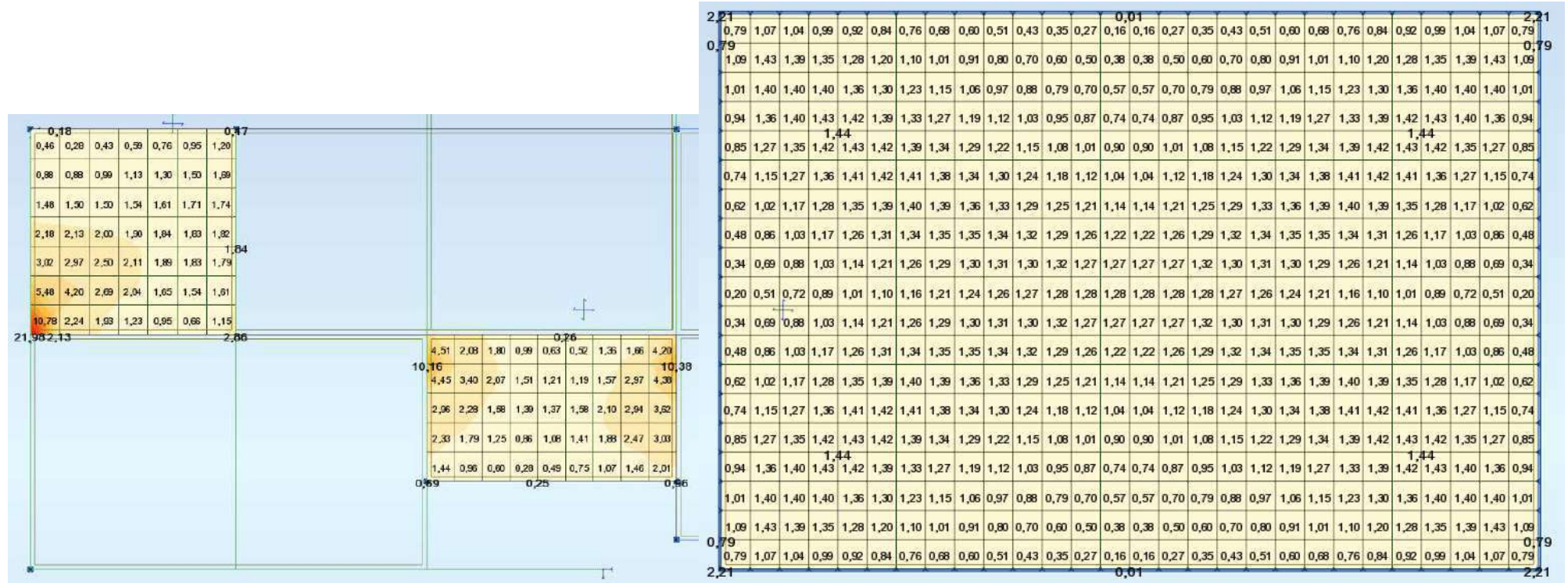
5.1.4 pav. Plokščių armavimas (Ay - apatinis) (ašys 3-5, A) (ašys 3-5, A)
