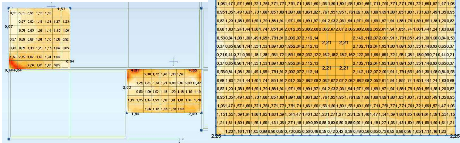
5.1.2 pav. Plokščių armavimas (Ax - apatinis) (ašys 3-5, A) (ašys 3-5, A)
