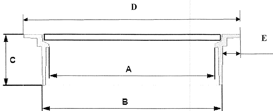
Pav. 1, Apžiūros šulinio liuko matmenys.
