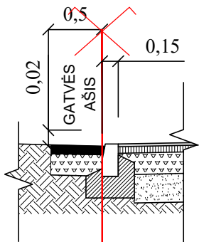
Nuovažos įrengimo detalė
