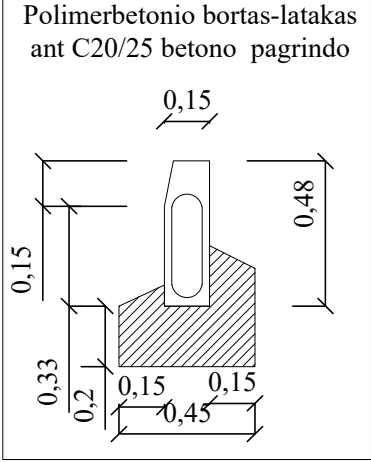
Nuovažos įrengimo detalė
