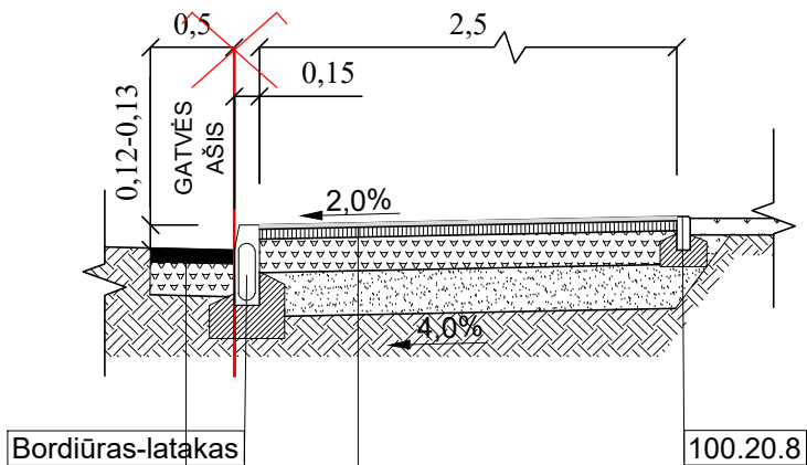
Skersinis profilis Nr. 2
