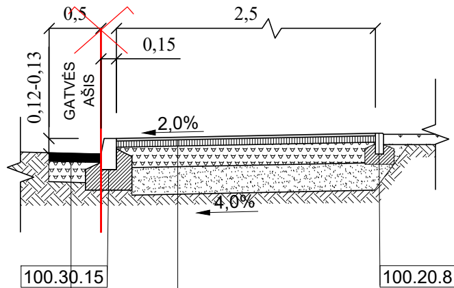
Skersinis profilis Nr. 1
