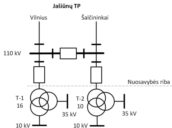
110/35/10 kV Jašiūnų TP principinė schema.
