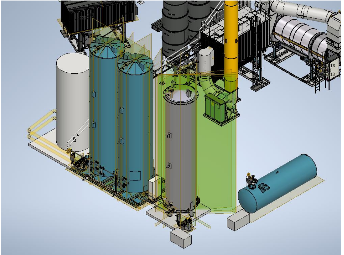
Pav. Nr. 1. Esamos ir planuojamos bitumo talpyklos vizualizacija
