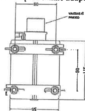
Antenų tvirtinimo adapterio pagrindiniai išmatavimai:
