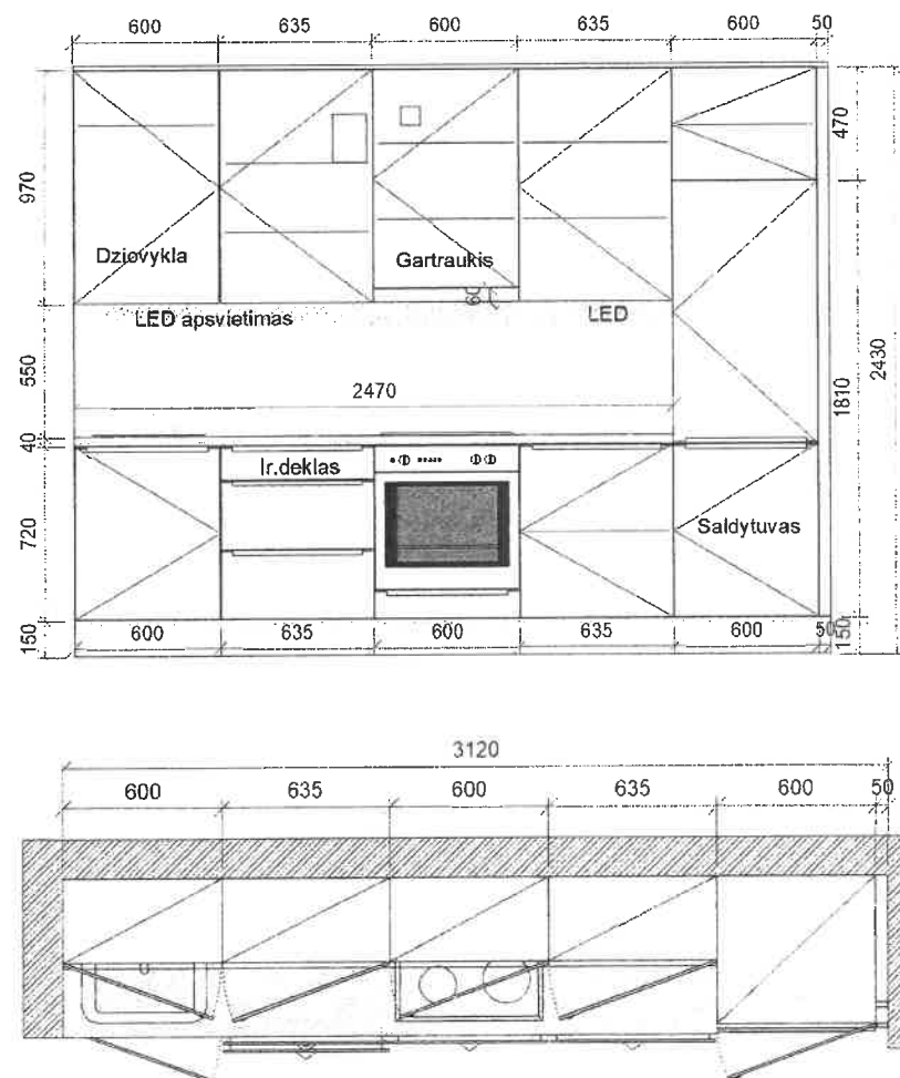
Brėžiniai
