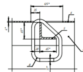
B - B 1:25
