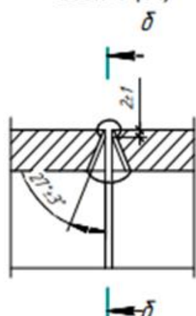
Узел 1 (1:1)
