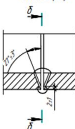
Узел 2 (1:1)
