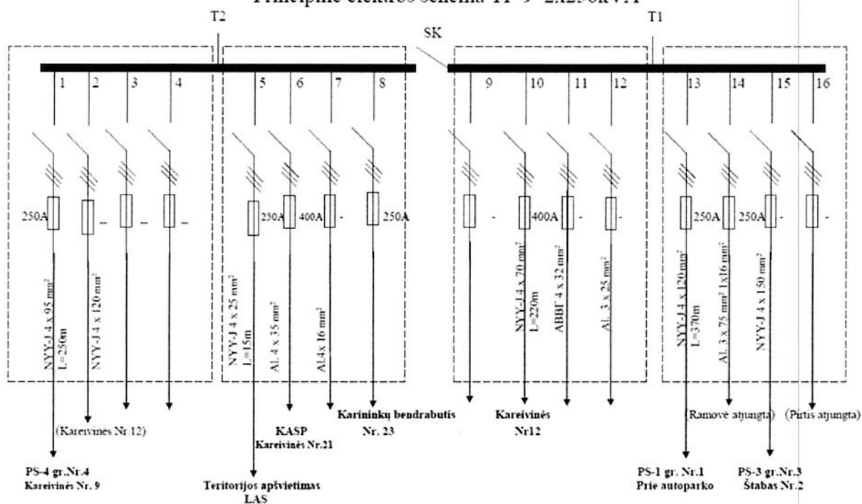
Principinė elektros schema TP-9 2x250kVA
