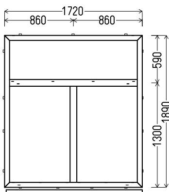
V2 (1vnt)
