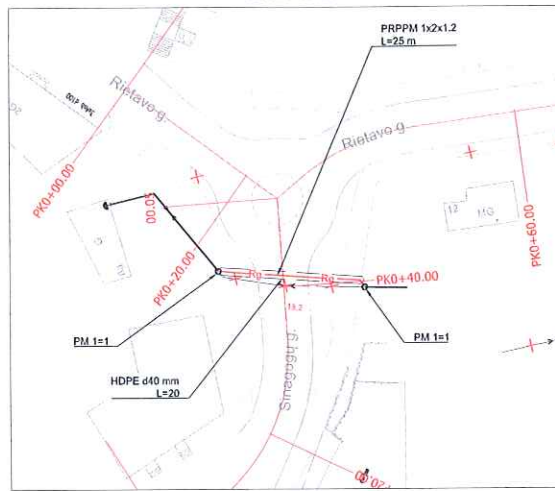
Schema Nr. 10
