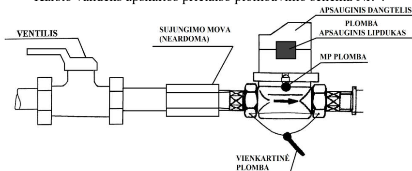
Karšto vandens apskaitos prietaiso plombavimo schema Nr. 4
