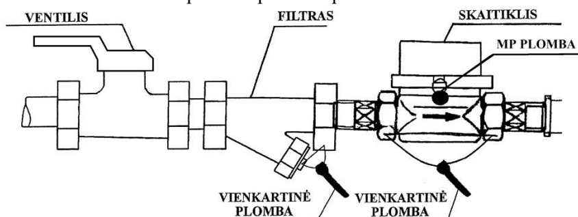
Karšto vandens apskaitos prietaiso plombavimo schema Nr. 2
