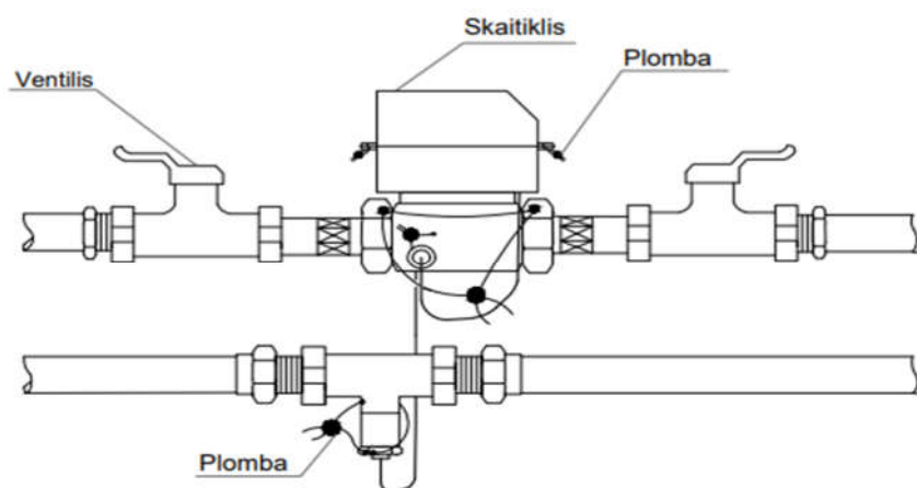
Šilumos apskaitos prietaiso plombavimo schema Nr. 1
