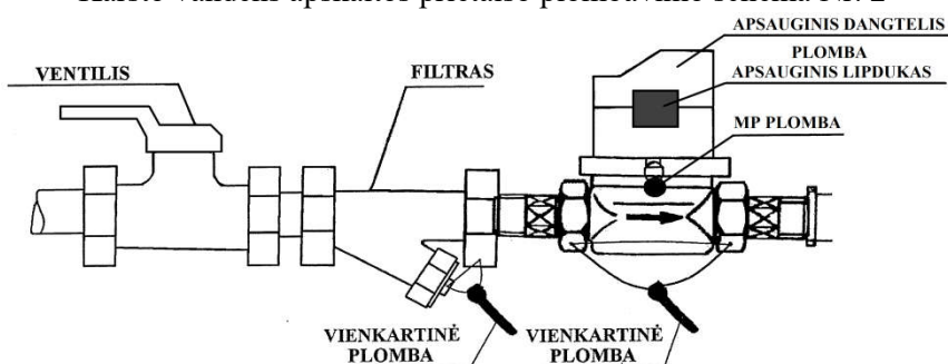
Karšto vandens apskaitos prietaiso plombavimo schema Nr. 3
