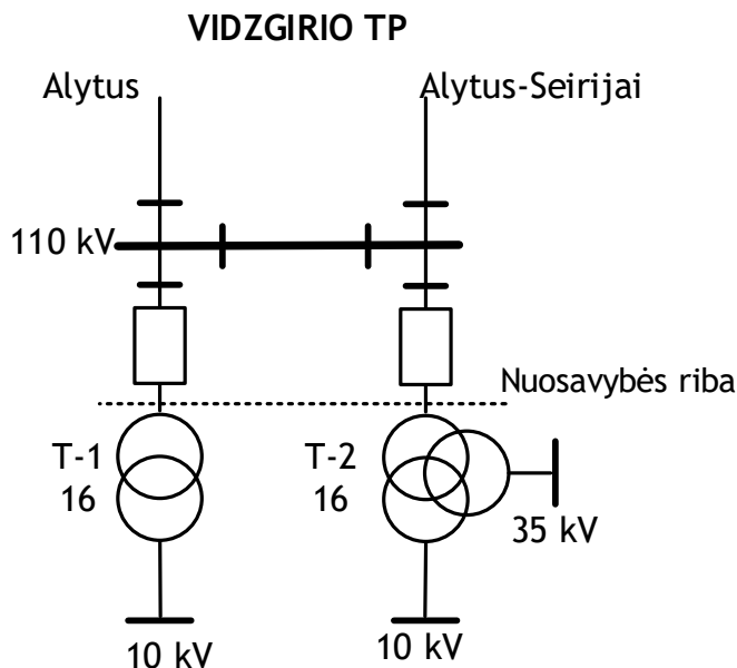
1 pav. 110/10 kV Vidzgirio TP 110 kV skirstyklos rekonstravimo principinė schema
