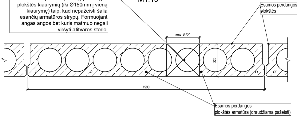
Pjūvis 1-1 M1:10
