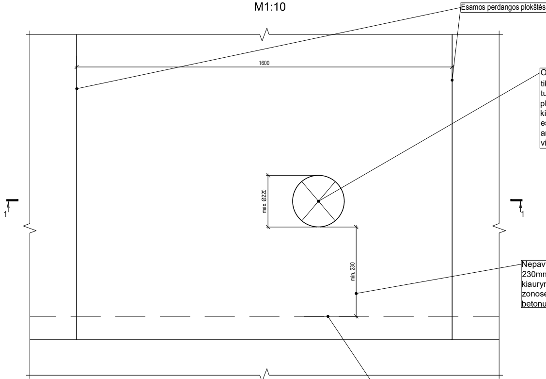
Pjūvis 1-1 M1:10
