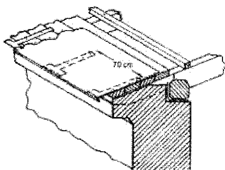
3 pav. Stoglovio juostos formavimas
