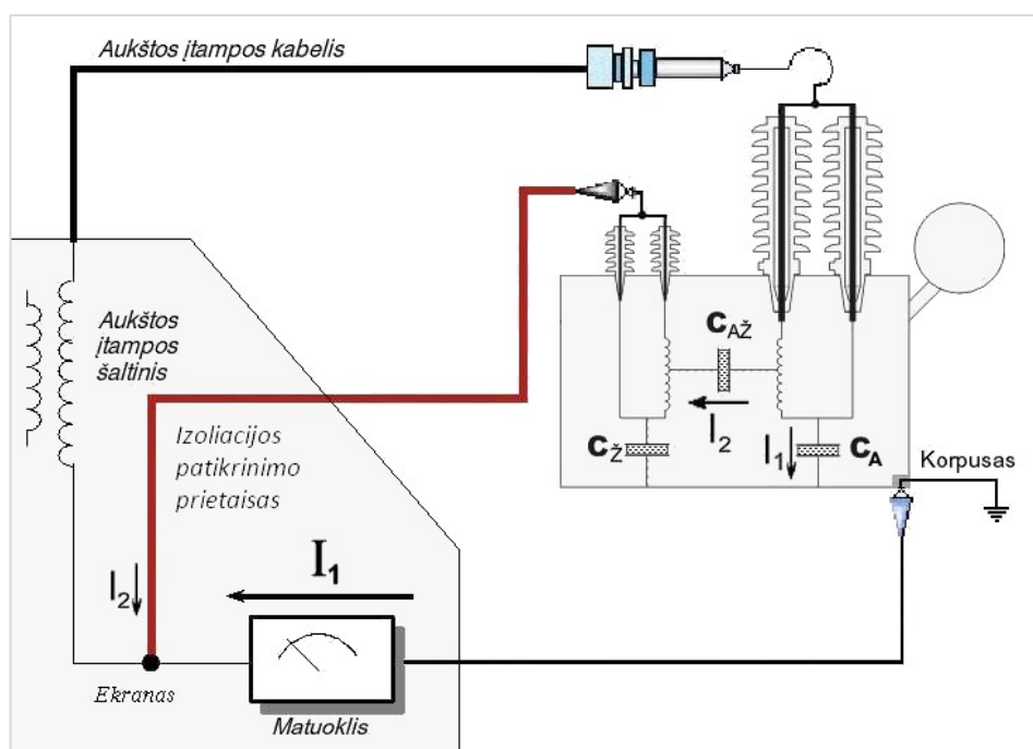
12 pav. Dviejų apvijų transformatorių, autotransformatorių apvijų izoliacijos dielektrinių nuostolių kampo \tan \delta ir talpio tarp aukštosios įtampos apvijos ir įrenginio korpuso patikrinimo schema ( A \rightarrow K )
