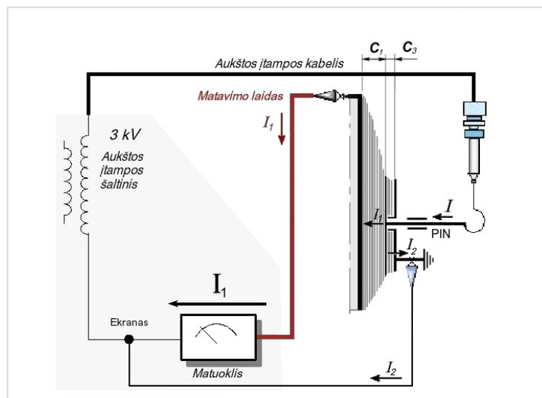
20 pav. Įvadų pagrindinės izoliacijos ( C_1 ) dielektrinių nuostolių kampo tgδ ir talpio papildoma matavimo schema (atvirkštinė)
