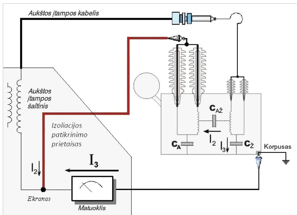
13 pav. Dviejų apvijų transformatorių, autotransformatorių apvijų izoliacijos dielektrinių nuostolių kampo tgδ ir talpio tarp žemosios įtampos apvijos ir įrenginio korpuso patikrinimo schema ( \check{Z} \rightarrow K )
