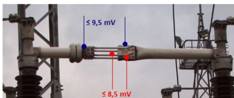
34 pav. SGF-123 tipo skyriklio kontaktų pereinamos varžos matavimas
