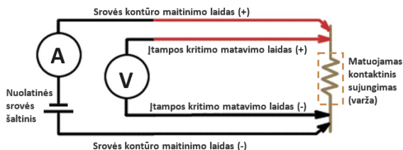
35 pav. Keturių laidų matavimo schema varžos nuolatinei srovei dydžiui nustatyti
