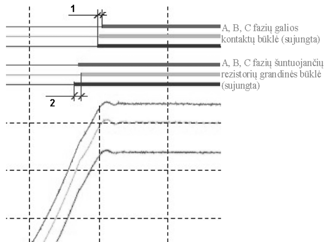
42 pav. Didelio alyvos tūrio jungtuvo įjungimo nevienalaikiškumo tikrinamas, kur: 1 - polių kontaktinių sistemų įjungimo nevienalaikiškumas; 2 - polių kameros šuntuojančių varžų įjungimo nevienalaikiškumas.
