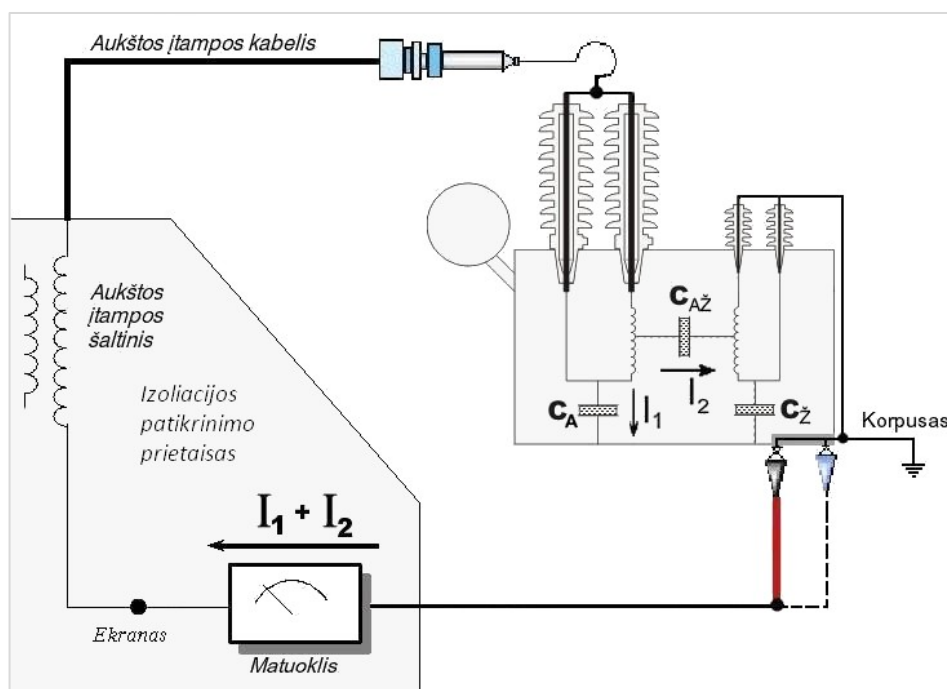
9 pav. Dviejų apvijų transformatorių, autotransformatorių apvijų izoliacijos dielektrinių nuostolių kampo tgδ ir talpio tarp aukštosios įtampos apvijos ir įžemintos žemosios įtampos apvijos patikrinimo schema ( A \rightarrow \check{Z}+K )
