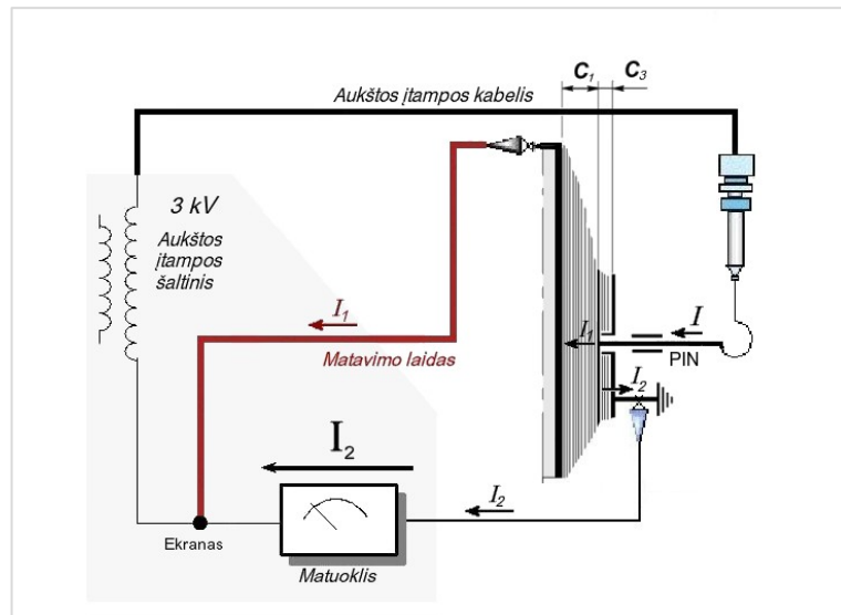
19 pav. Įvadų paskutinio izoliacijos sluoksnio ( C_3 ) dielektrinių nuostolių kampo tgδ ir talpio matavimo schema
