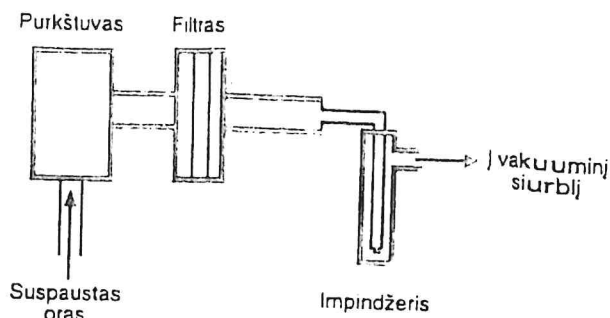
1 pav. Bandymų sistemos schema
