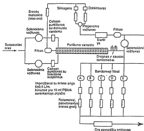
1 pav. Filtro bandomasis modelis (Hendersono įtaisas)
