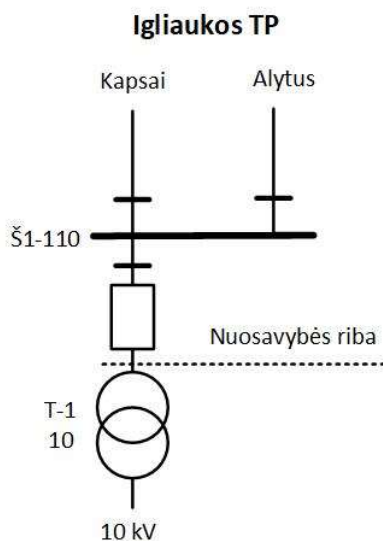
1 pav. 110/10 kV Igliaukos TP rekonstravimo principinė schema
