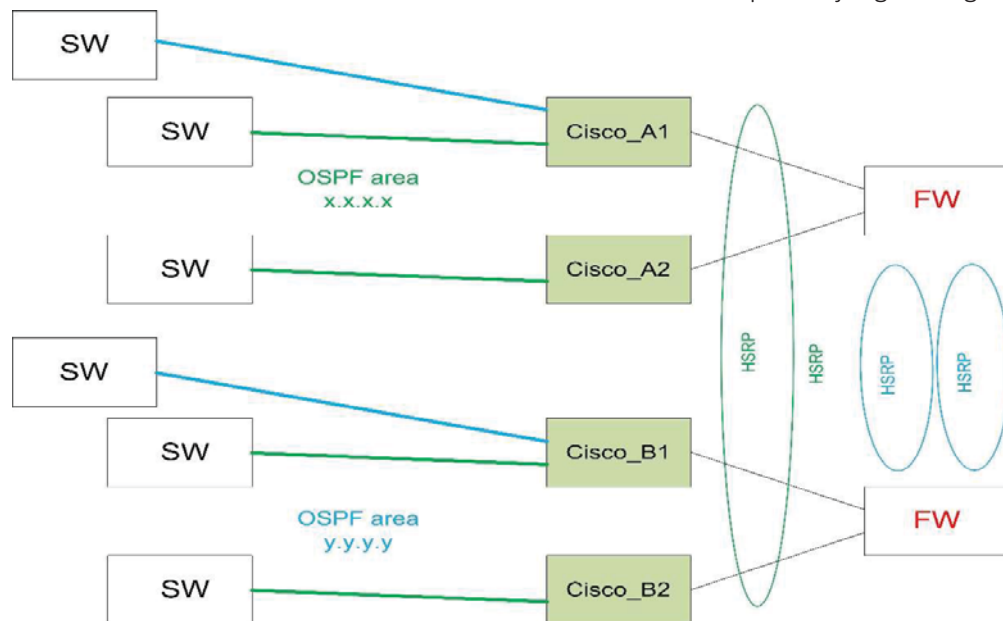
1 pav. Sujungimo loginė schema
