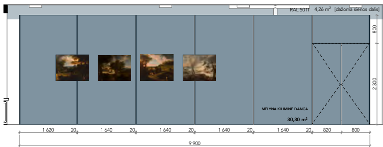
IŠKLOTINĖ 2.01_D M1:50
