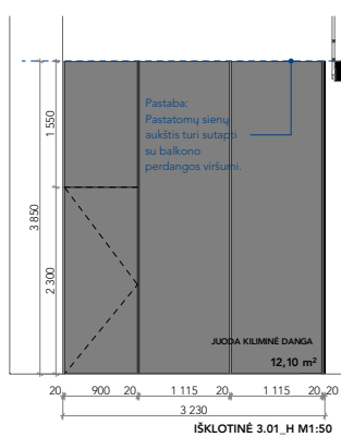
IŠKLOTINĖ 3.01_H M1:50
