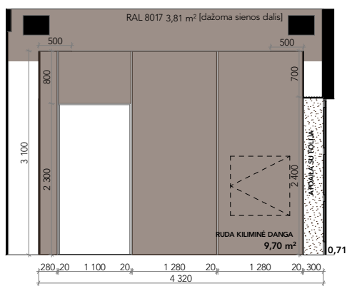
IŠKLOTINĖ 2.05_D M1:50
