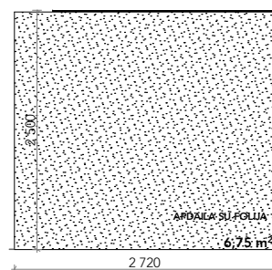
IŠKLOTINĖ 2.03_H M1:50
