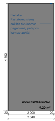
IŠKLOTINĖ 3.01_G M1:50
