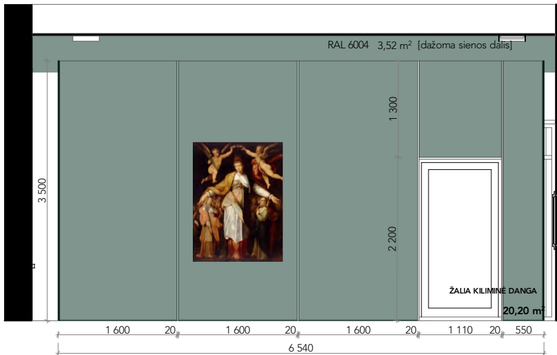
IŠKLOTINĖ 3.02_D M1:50
