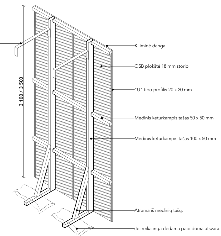
ANTRO AUKŠTO SIENŲ KONSTRUKTYVINĖ SCHEMA
