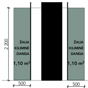
IŠKLOTINĖ 3.03_F1 M1:50
