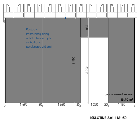
IŠKLOTINĖ 3.01_I M1:50
