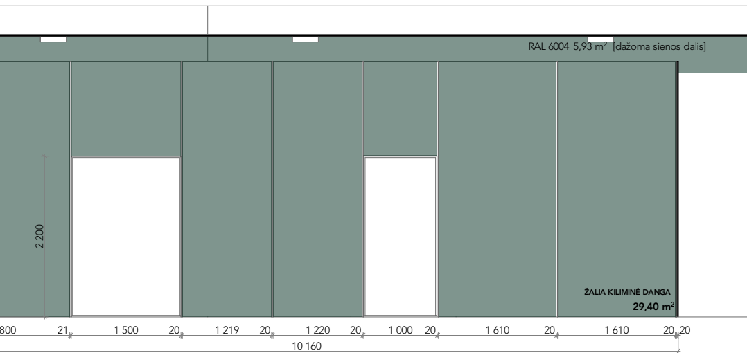
IŠKLOTINĖ 3.03_C M1:50
