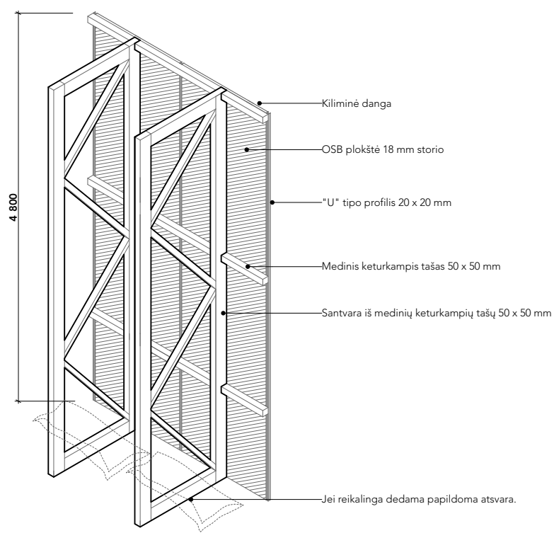
TREČIO AUKŠTO SIENŲ KONSTRUKTYVINĖ SCHEMA
