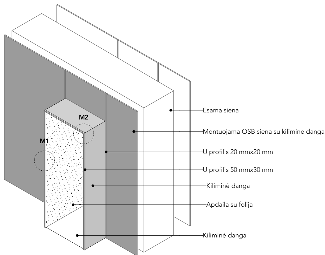
ARKOS AKSONOMETRINĖ SCHEMA
