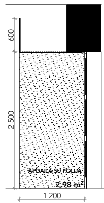
IŠKLOTINĖ 2.04_E M1:50
