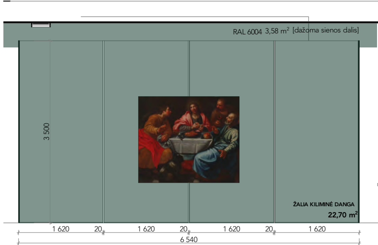
IŠKLOTINĖ 3.02_B M1:50
