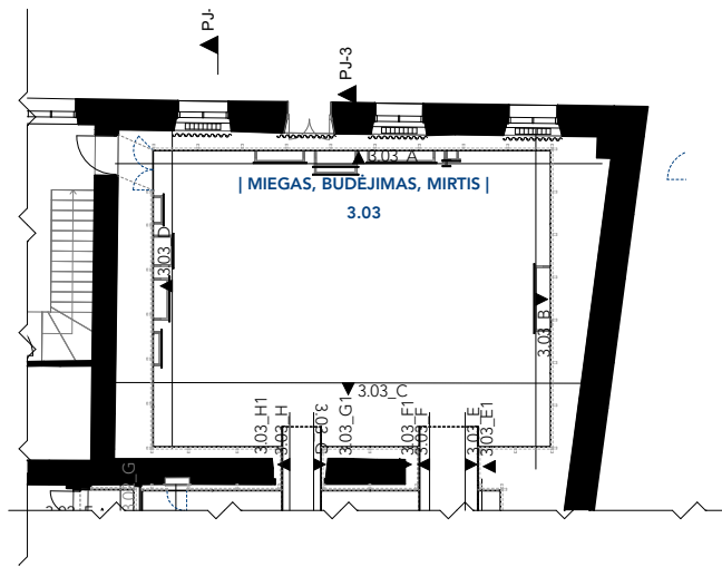
PATALPOS PLANAS M1:150
