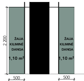
IŠKLOTINĖ 3.03_G1 M1:50
