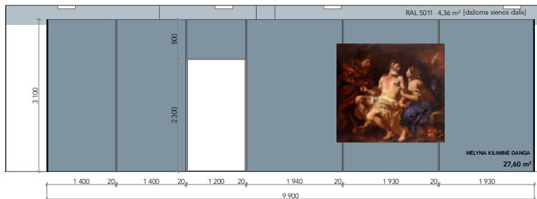
IŠKLOTINĖ 2.01_B M1:50
