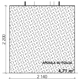
IŠKLOTINĖ 3.03_G M1:50
