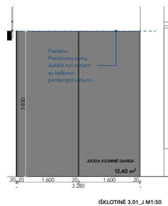
IŠKLOTINĖ 3.01_J M1:50
