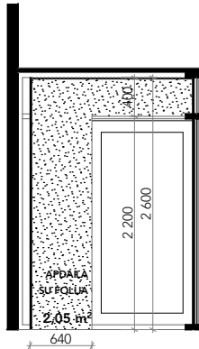
IŠKLOTINĖ 3.02_G M1:50
