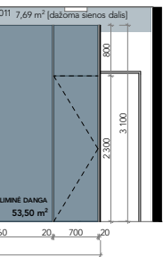
IŠKLOTINĖ 2.01_A M1:50
