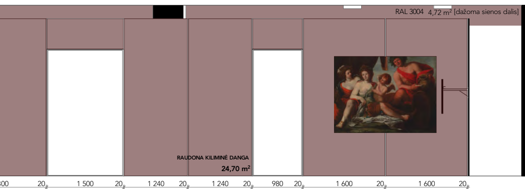
IŠKLOTINĖ 2.03_C M1:50
