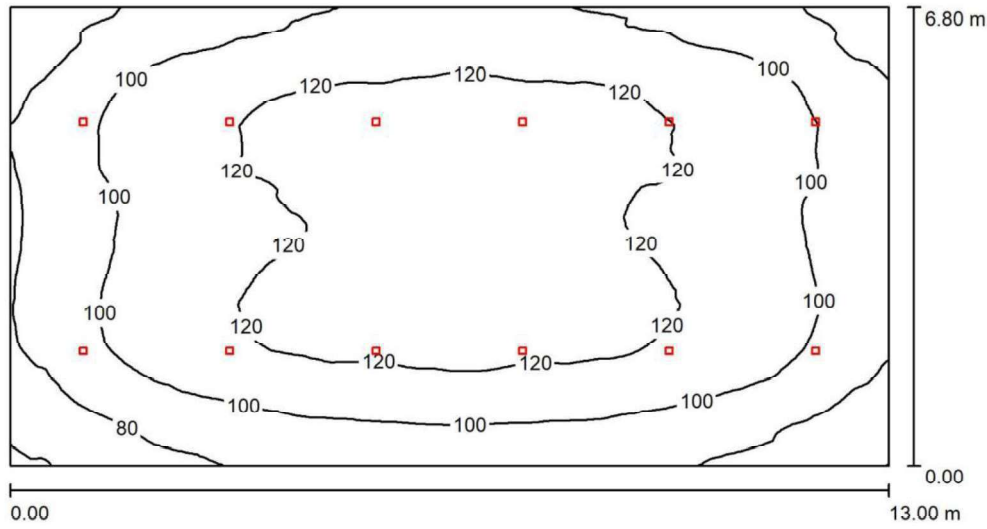
Apšvietos schema:
