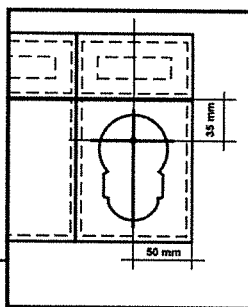
Muitininko ženklų tvirtinimo skylutė (ženklų matmenys 85 x 55 mm)
