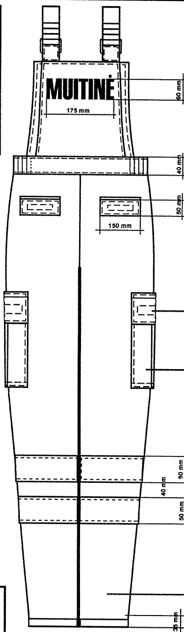
Muitininko ženklų tvirtinimo skylutė (ženklų matmenys 85 x 55 mm)
