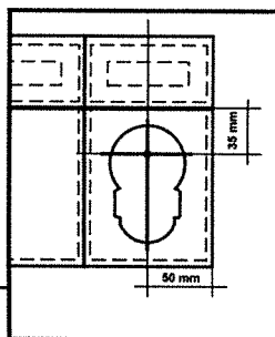
Muitininko ženklo tvirtinimo skylutė (ženklų matmenys 85 x 55 mm)
