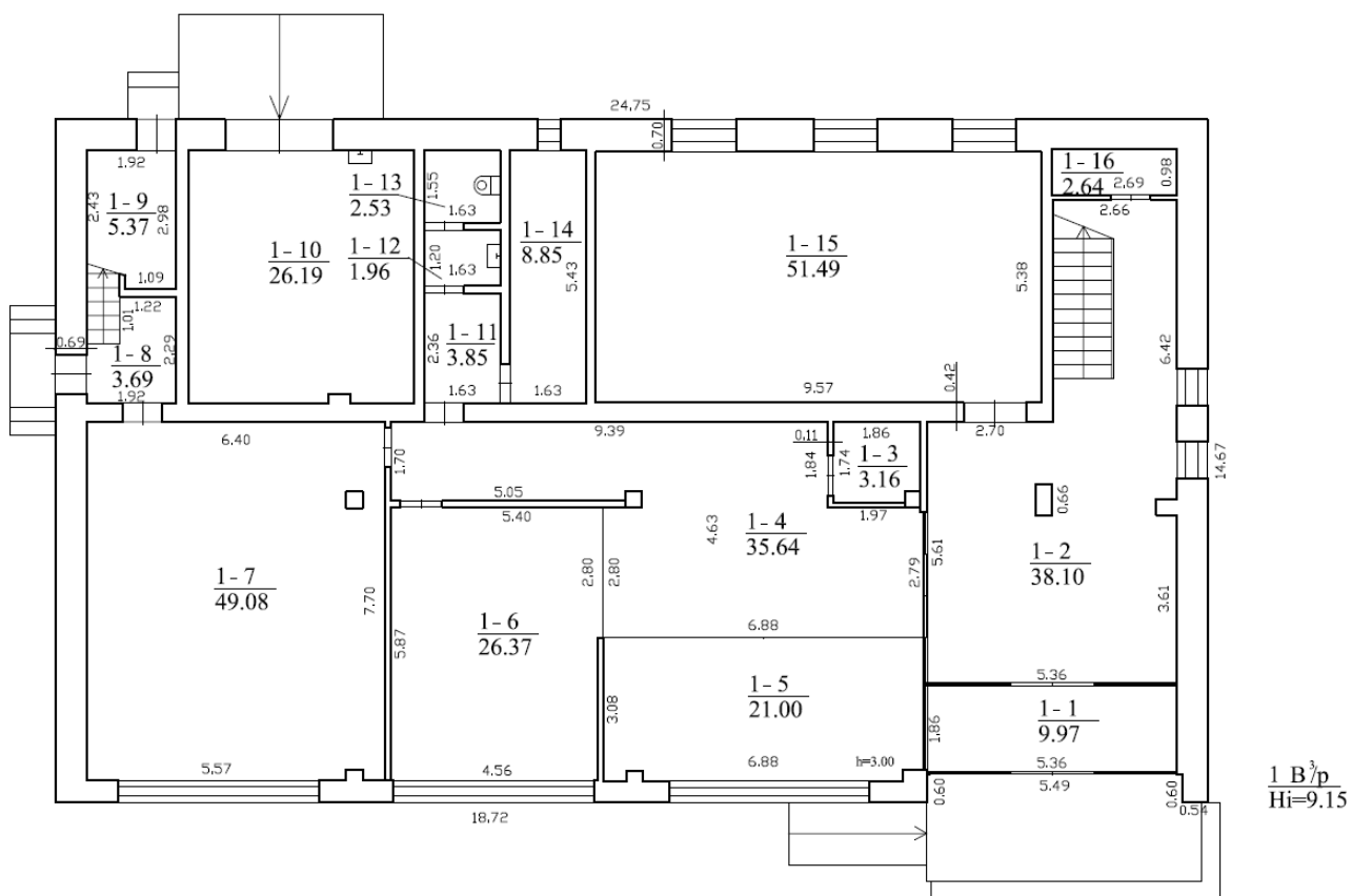
1 aukšto planas
