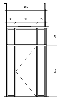
SN-207 PVC pertvara
