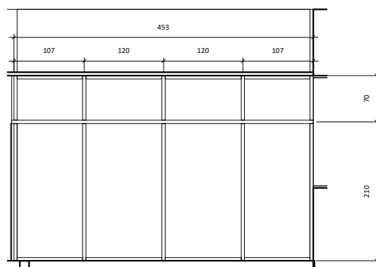
SN-208 PVC pertvara
