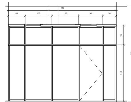
SN-117 Aliuminio pertvara
