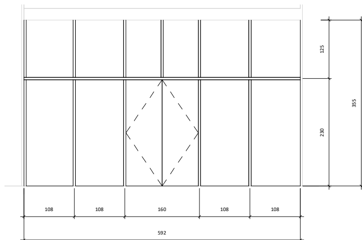
SN-114 Aliuminio pertvara
