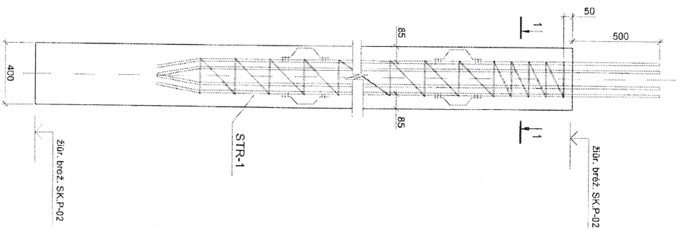
Gręžinis pamatas GP-1
