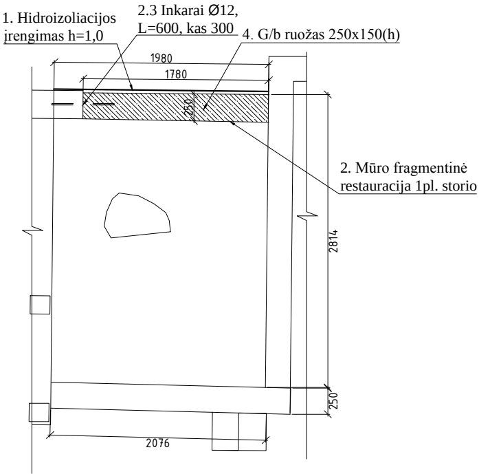
Kapo planas M1:50
