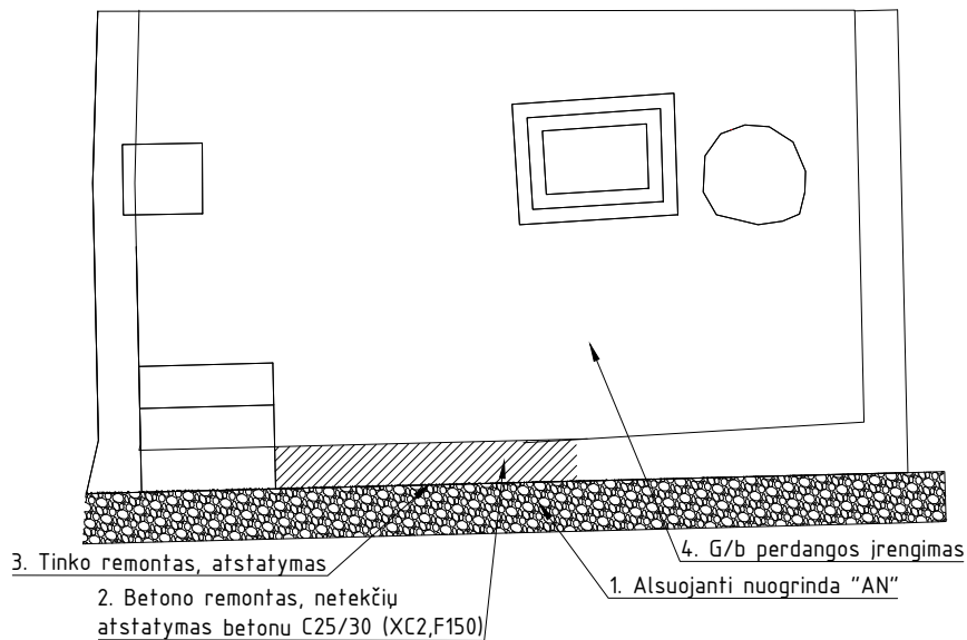
Alsuojanti nuogrinda "AN" M1:20
