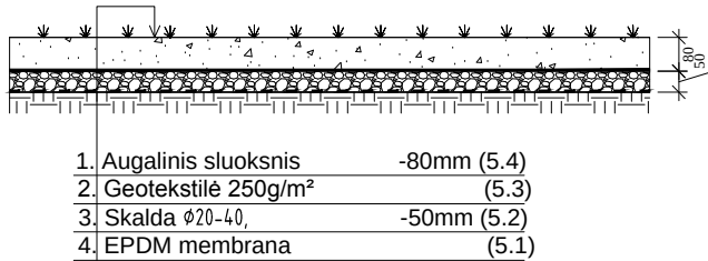
Drenažinis sluoksnis "DR" M1:20
