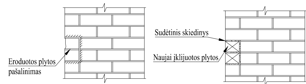
Mūro fragmentinēs restaurācijas detālē "MR1" M 1:20
