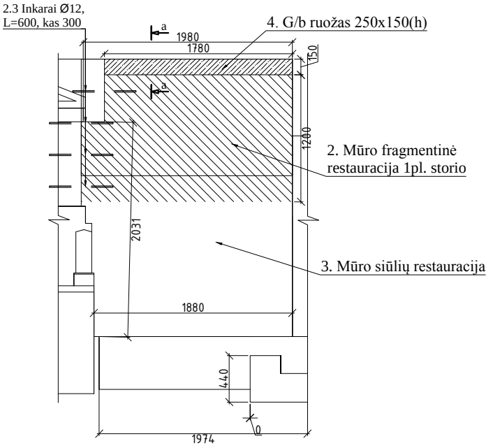
Siūlių restauracijos detalė "MR2" M 1:20
