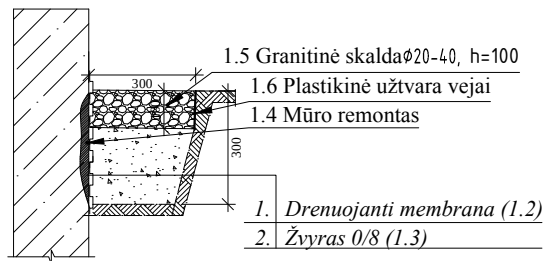
Alsuojanti nuogrinda "AN" M1:20
