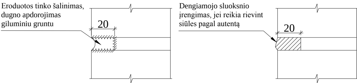
Siūlių restauracijos detalė "MR2" M 1:20
