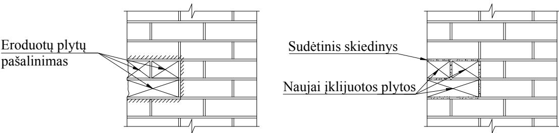
Mūro fragmentinės restauracijos detalė "MR1" M 1:20
