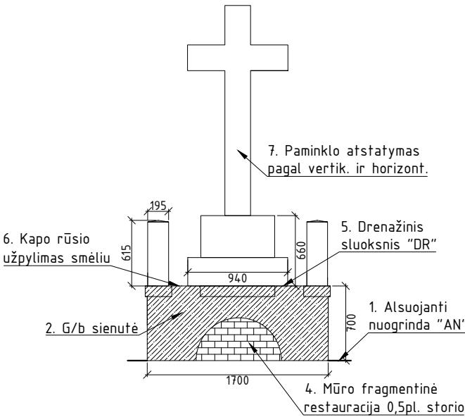
Priekinis fasadas M1:50
