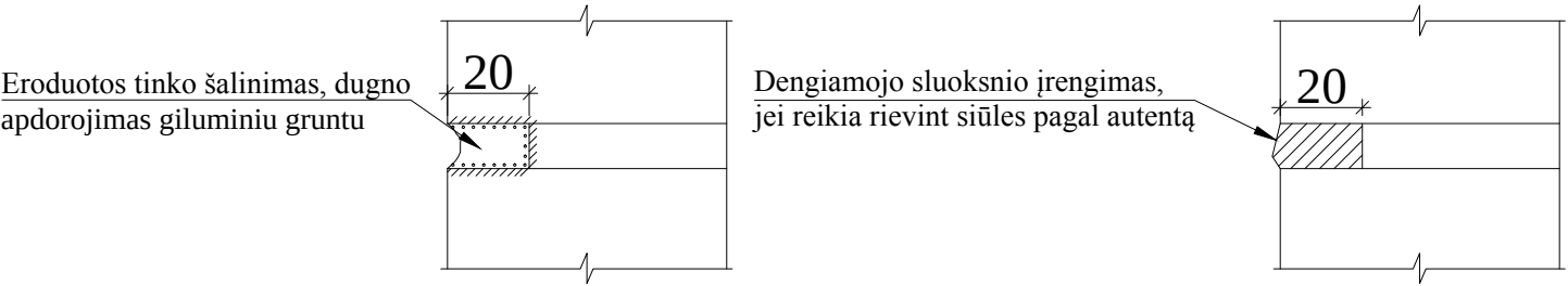
Siūlių restauracijos detalė "MR2" M 1:20
