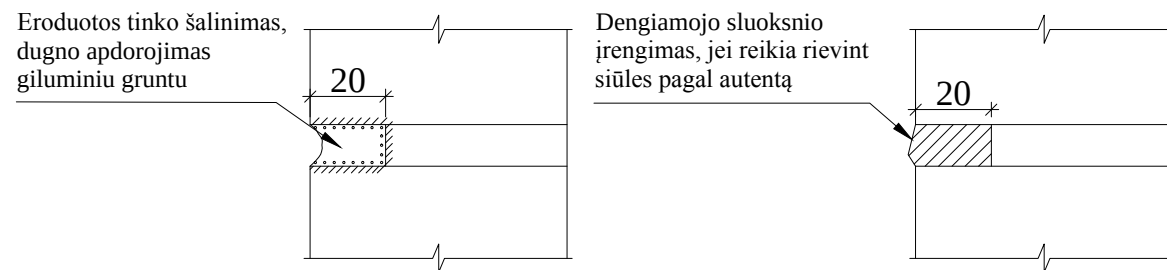
Siūlių restauracijos detalė "MR2" M 1:20
