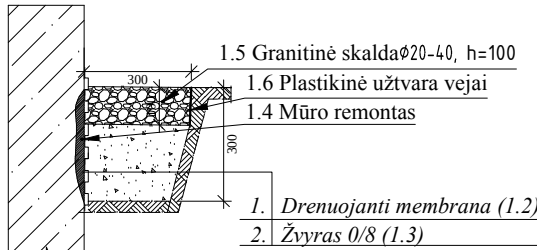
Alsuojanti nuogrinda "AN" M1:20
