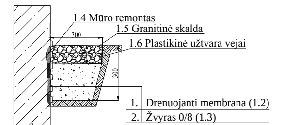
ALSUOJANTI NUOGRINDA "AN" M1:20
