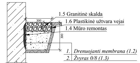
Alsuojanti nuogrinda "AN" M1:20
