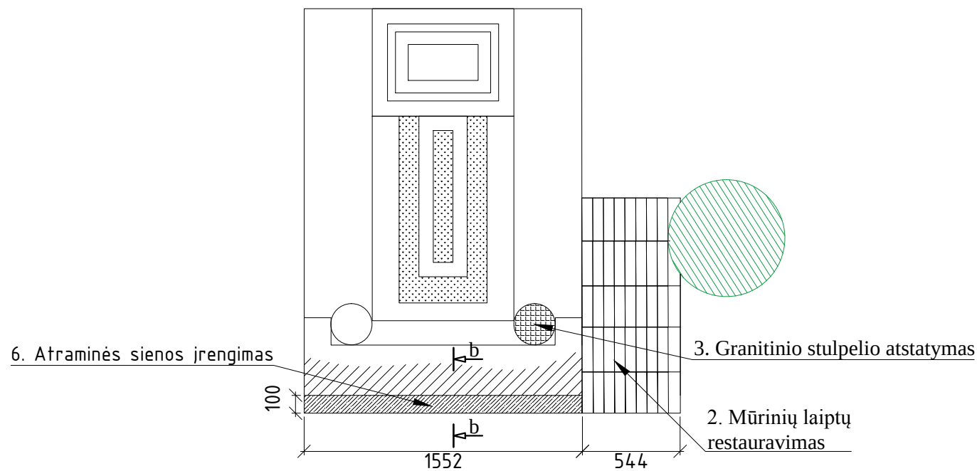
Kapo planas M1:30
