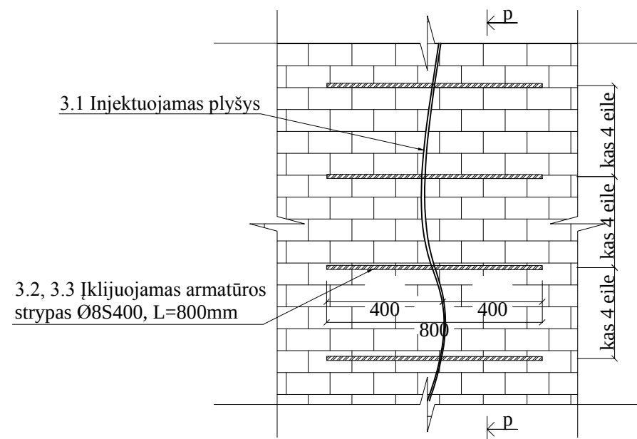
Plyšių injekavimo ir susiuvimo detalė "PL" M 1:20
