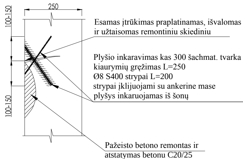
Pjūvis a-a M1:10
