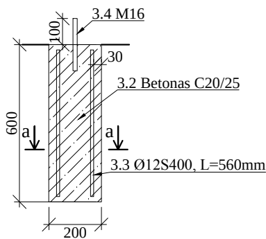
PAMATAS STULPELIUI "P" M1:20
