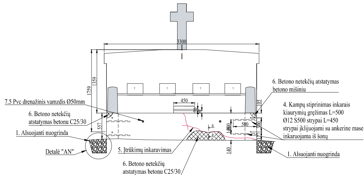
Pjūvis a-a M1:10
