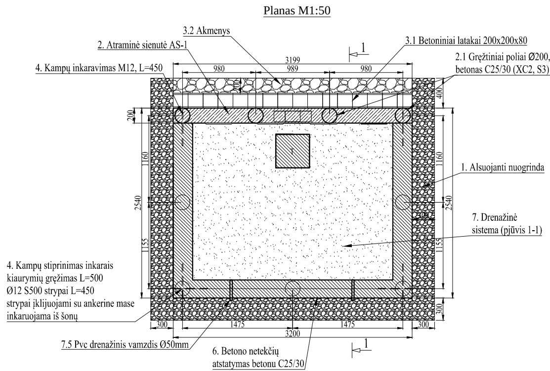
Priekinis fasadas M1:50
