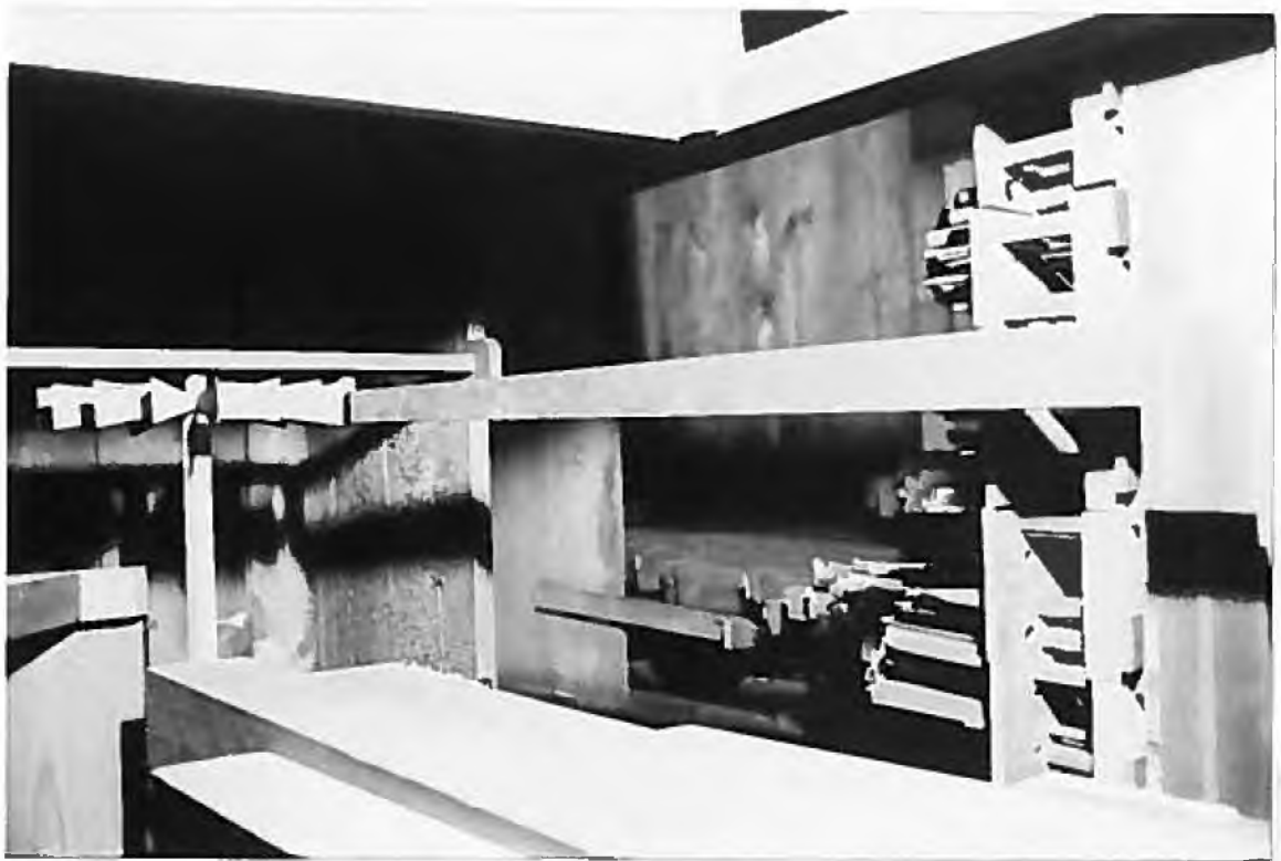
Nr. 19 Pavadinimas II manualo oro dėžė ir Žvaigždinių varpelių įrenginio malūnėlis su ortakiu Fotografavo R. Gučas Data ~1990 m.
