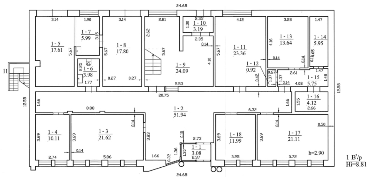
Pirmo aukšto planas adresu Livonijos g. 10, Joniškis
