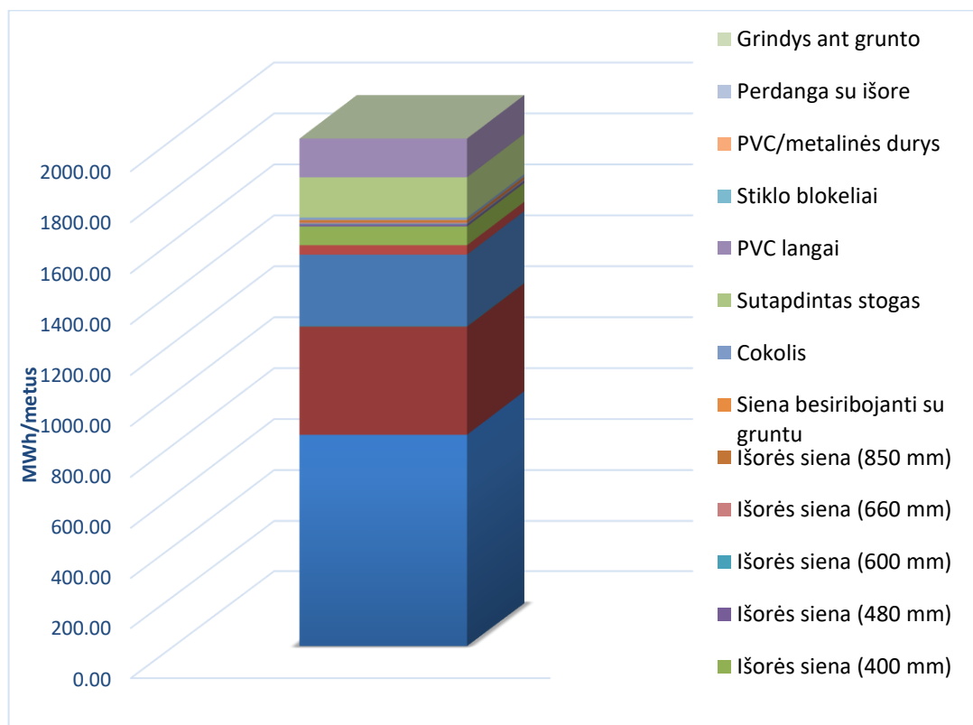
7 pav. Išorinių atitvarų nuostoliai bendrame pastato šilumos nuostolių balanse
