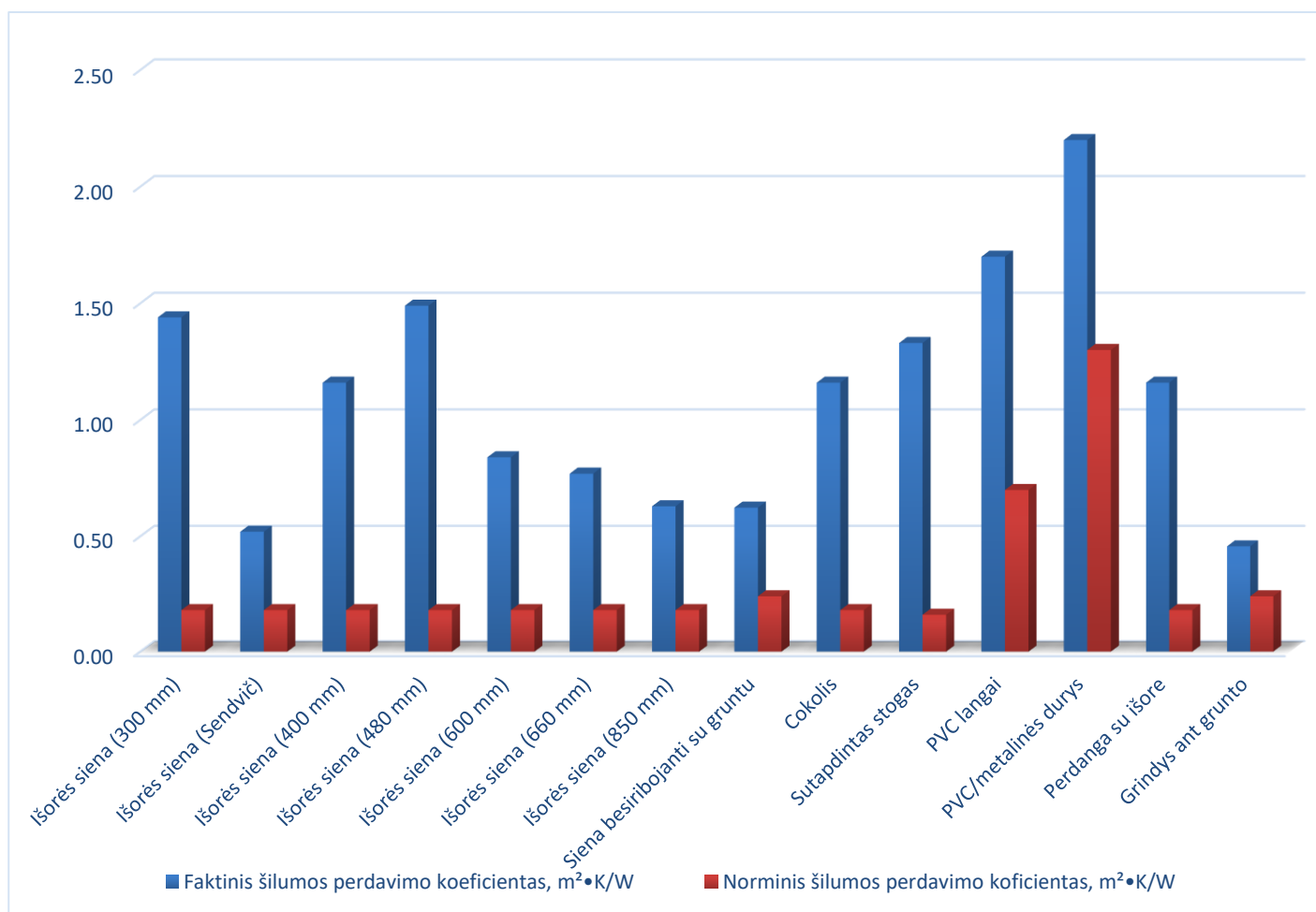
6 pav. Faktiniai ir norminiai šilumos perdavimo koeficientai.
