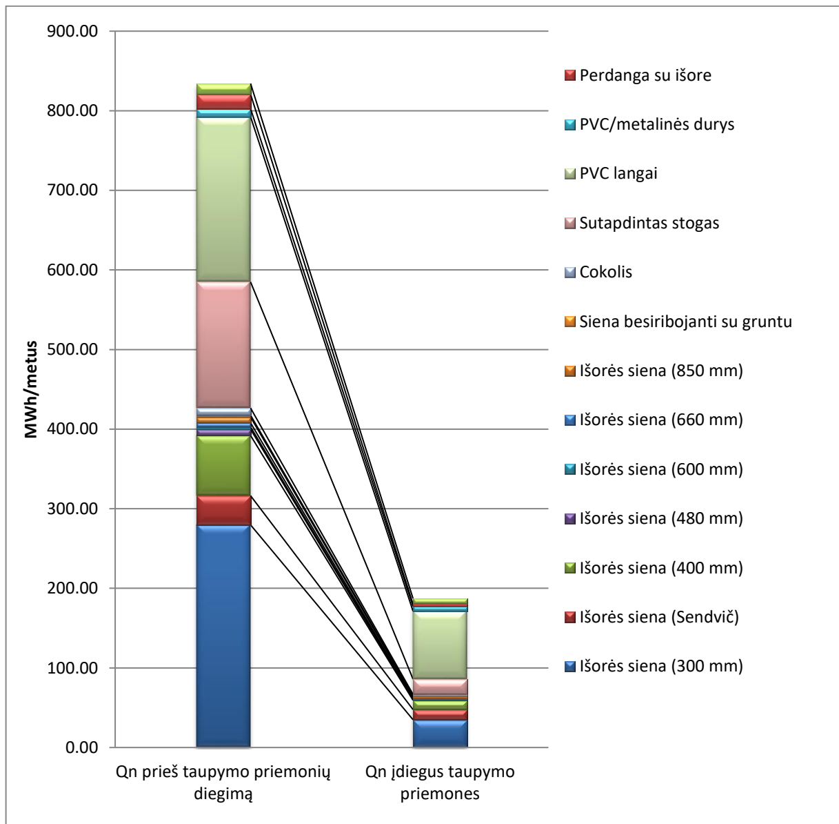
8 pav. Q_n prieš ir po taupymo priemonių diegimą
