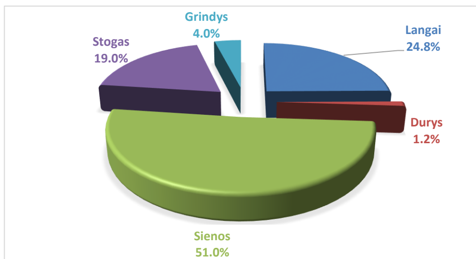
4 pav. Šilumos nuostoliai atitvarose
