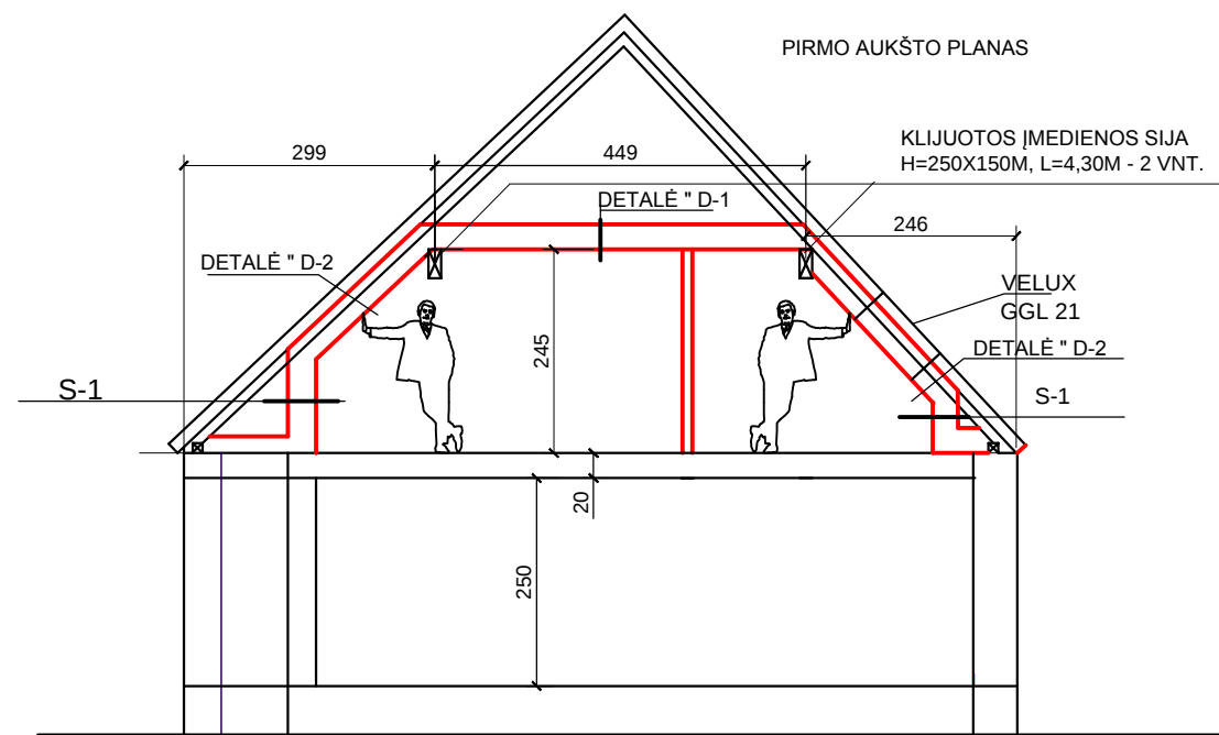
PJŪVIS 1-1
