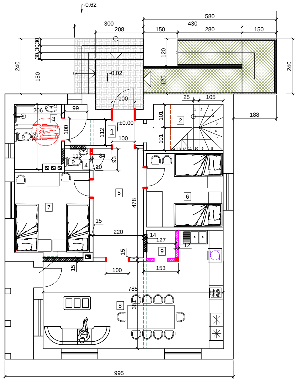
PIRMO AUKŠTO PLANAS SU BALDŲ IŠDĖSTYMU
