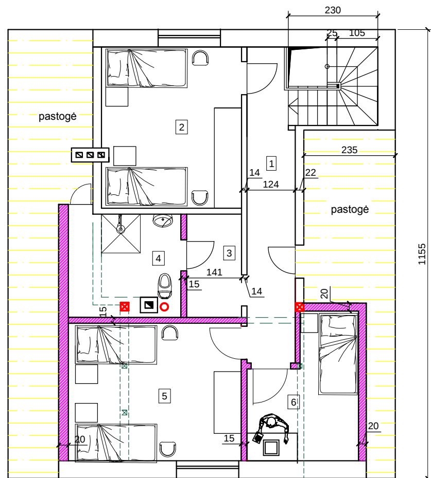
MANSARDOS PLANAS SU BALDŲ IŠDĖSTYMU
