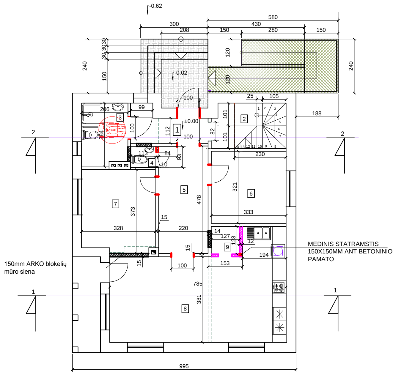
PIRMO AUKŠTO PLANAS
