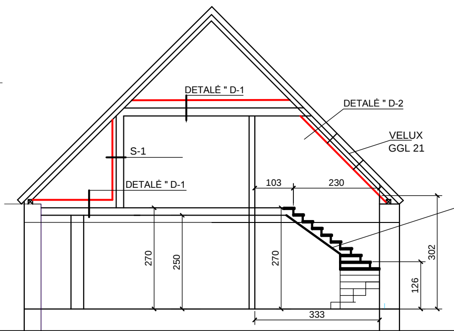
PJŪVIS 2-2
