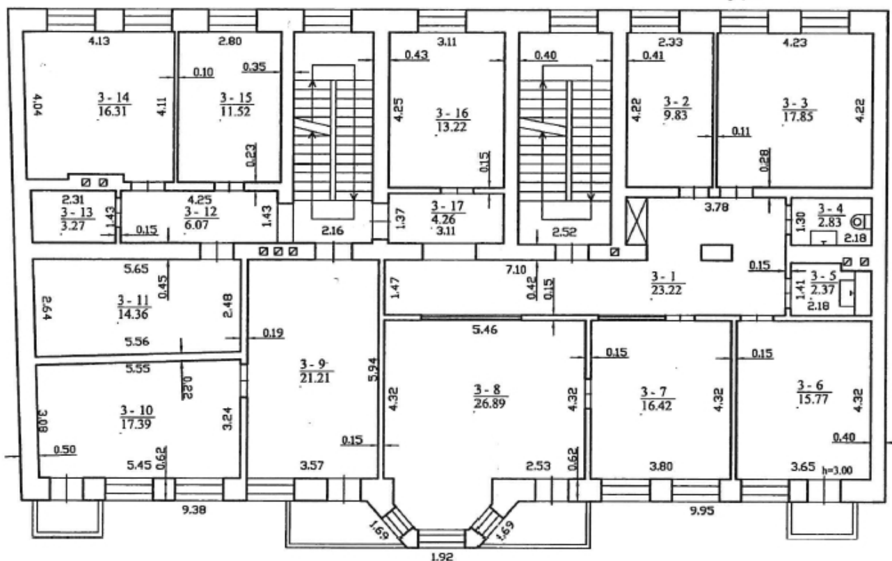
Tilžės g. 152, Šiauliuose trečio aukšto planas
