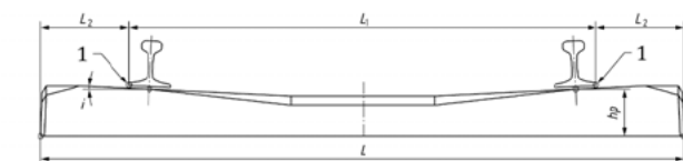
1 priedas. Tipinė vienblokių gelžbetoninio pabėgio schema
