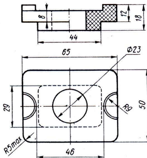
1 brėžinys. Izoliacinė įvorė
