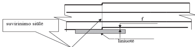
5 priedas. Laiptelio matavimas pade
