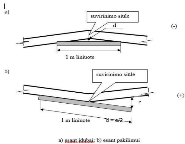
4 priedas. Suvirintų sandūrų nelygumų tikrinimas darbinėje briaunoje
