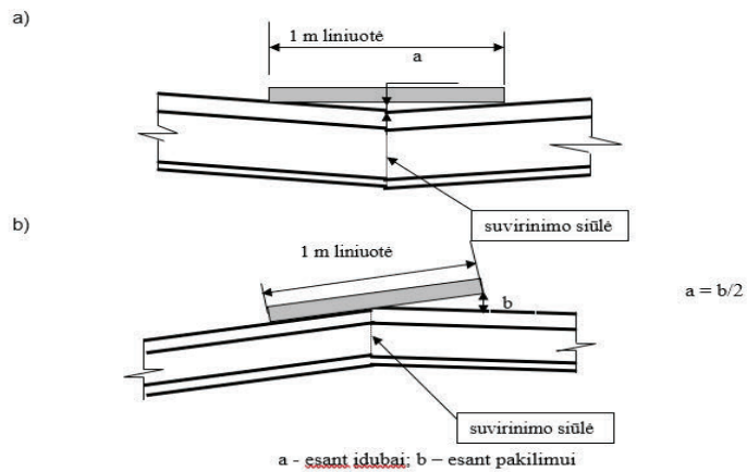
2 priedas. Suvirintų sandūrų nelygumų tikrinimas važiavimo paviršiuje
