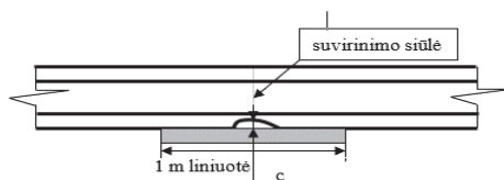
3 priedas. Nelygumų pado pakraščiuose matavimas
