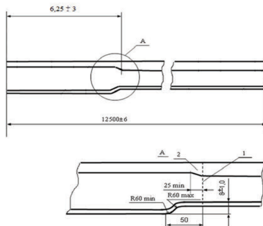
1 – suvirinimo sandūra; 2 – bėgio galvutės apdirbimo zona
