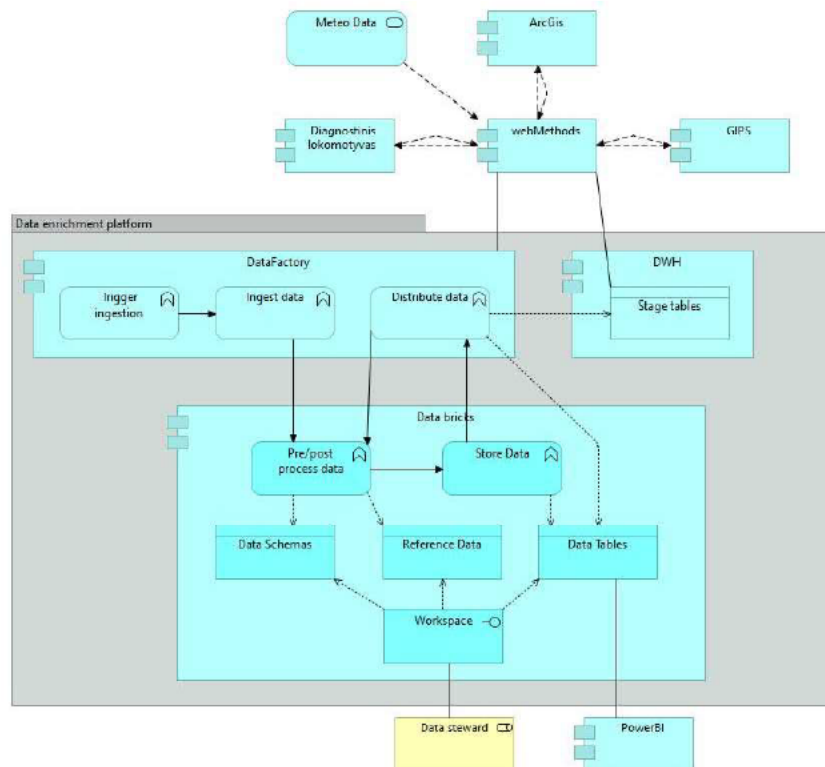
Paveikslas Nr. 2 Pavyzdinė, bandomojo modelio architektūra.
