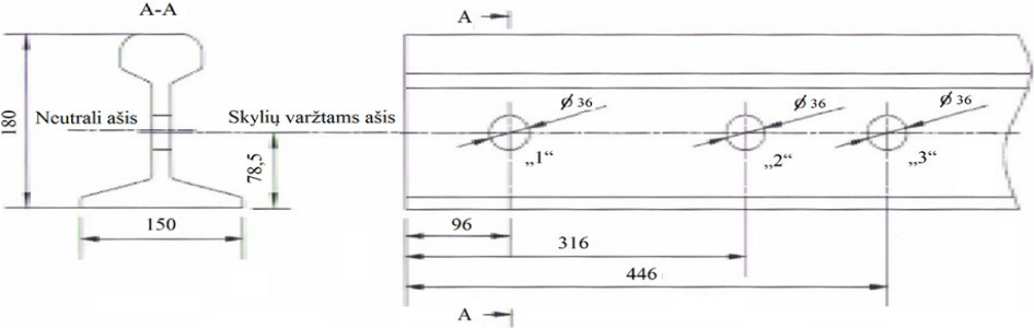
1 priedas. R65 tipo bėgyje skylių gręžimo nužymėjimo schema
