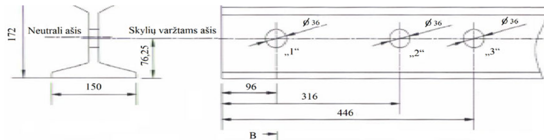
1 priedas. UIC60 (60E1) tipo bėgyje skylių gręžimo nužymėjimo schema
