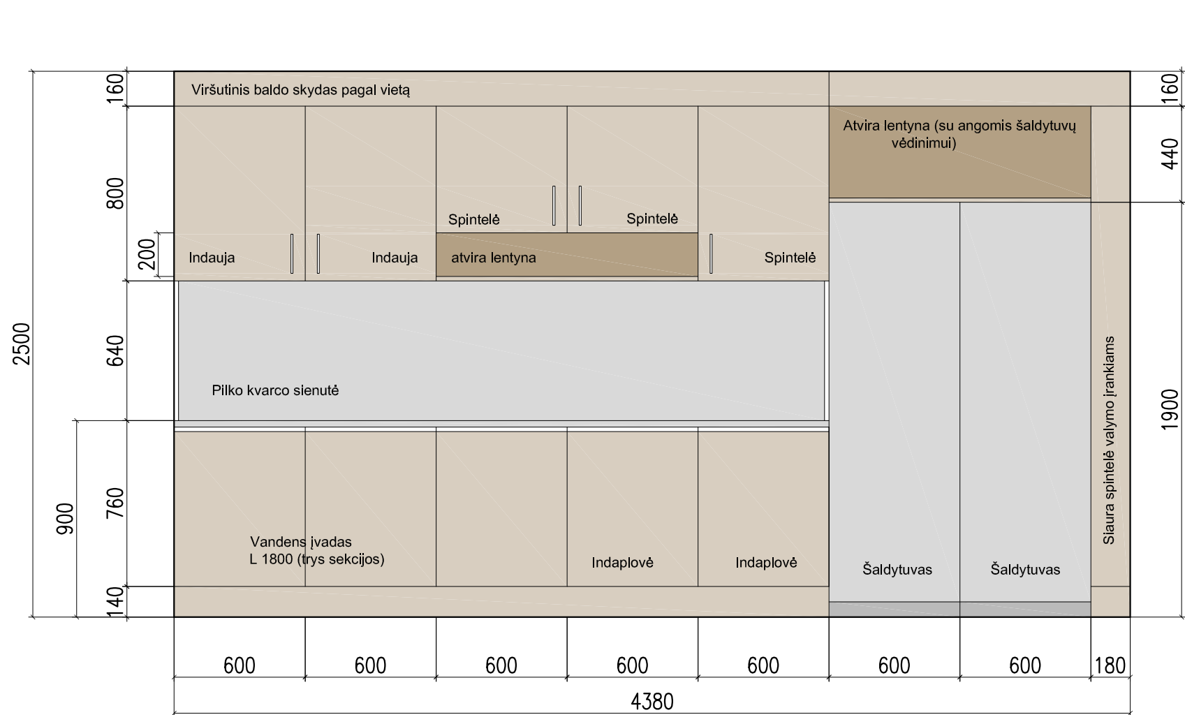
Virtuvės baldo vaizdas iš priekio
