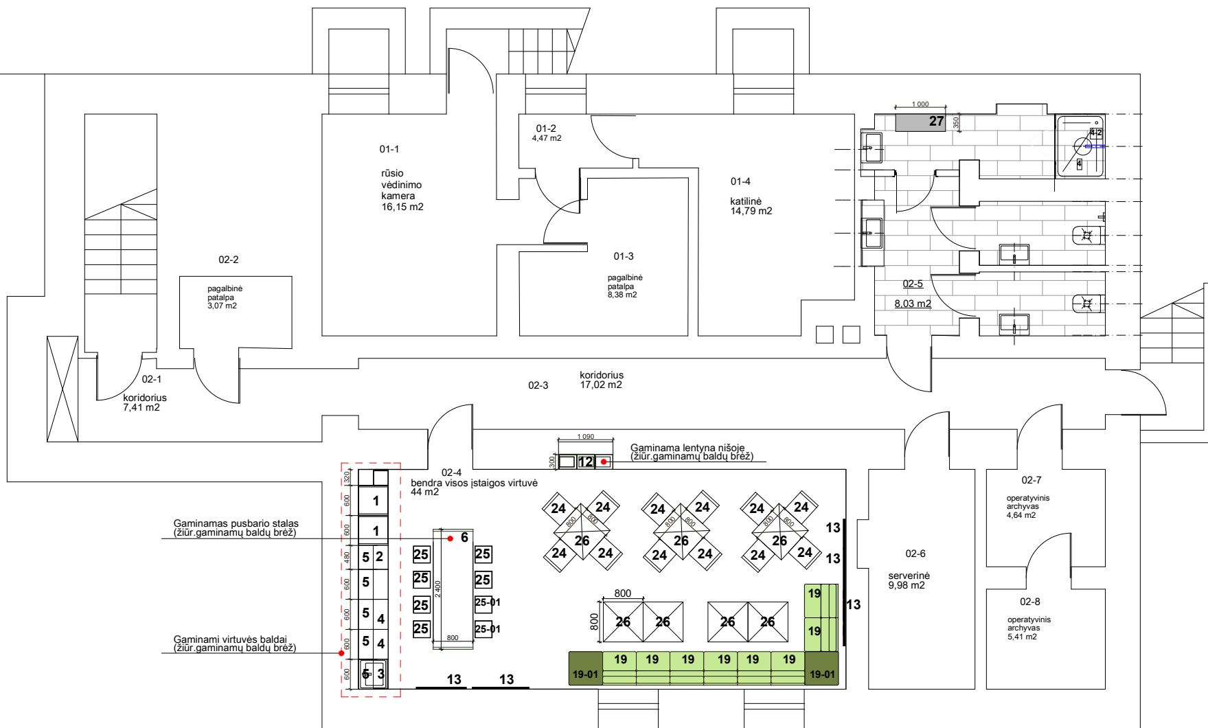
Rūsio planas
