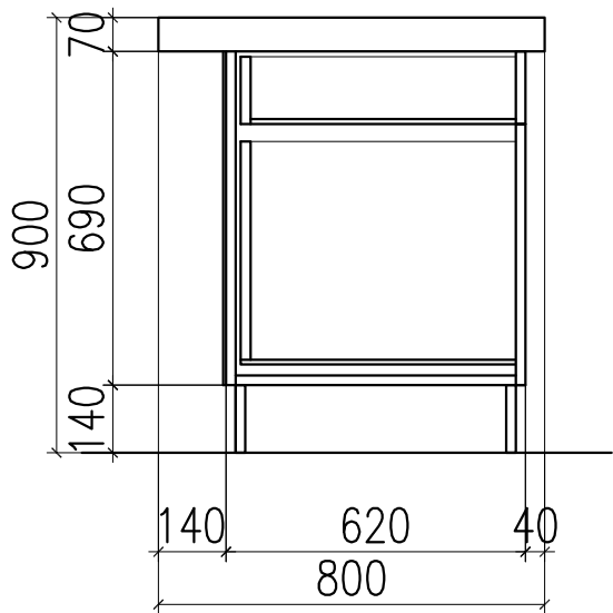
Pjūvis 2-2
