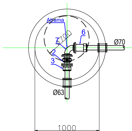
ŠULINYS VS1-4
