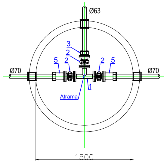
ŠULINYS VS1-4
