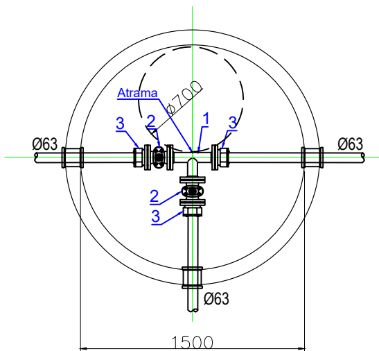
ŠULINYS VS1-3
