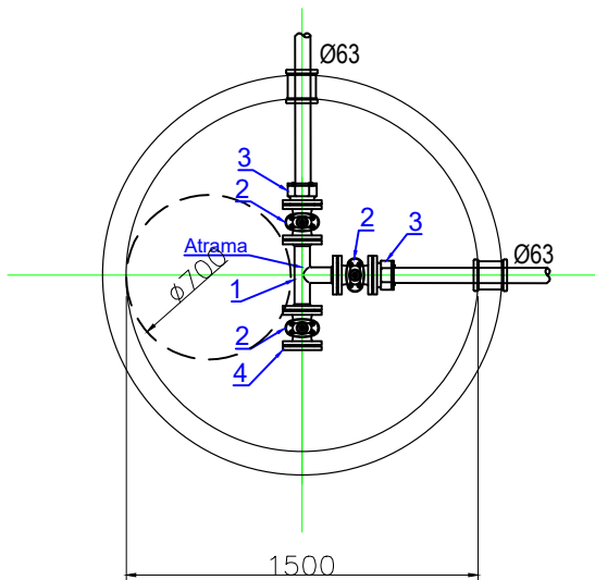
ŠULINYS VS1-3
