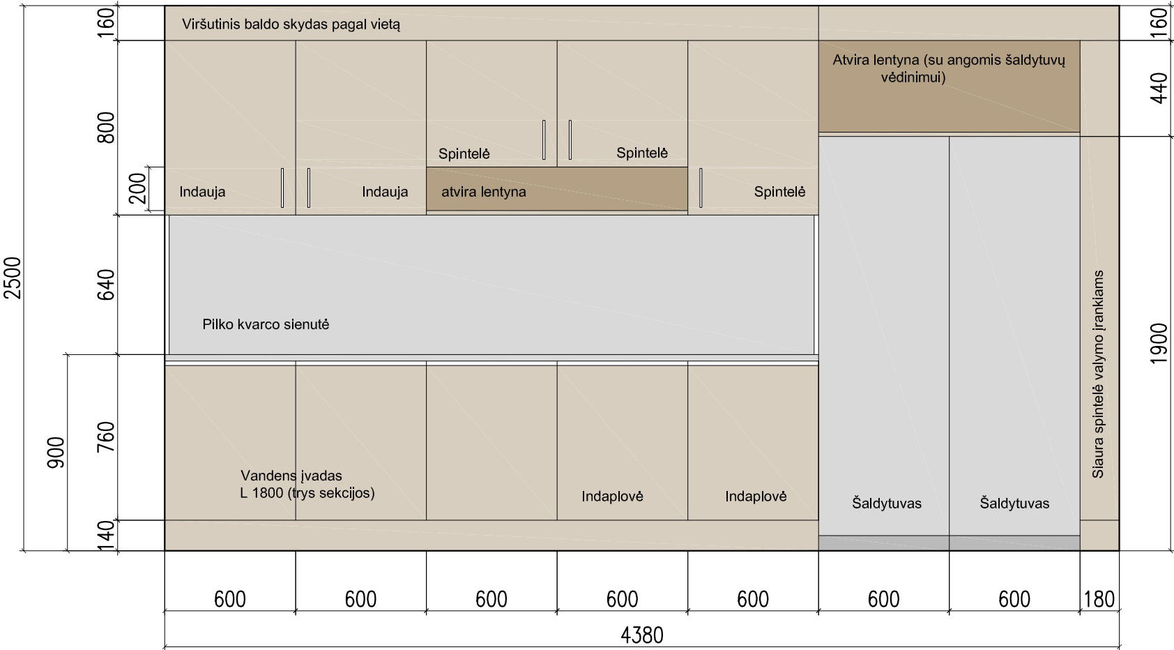
Virtuvės baldų vaizdas iš priekio
