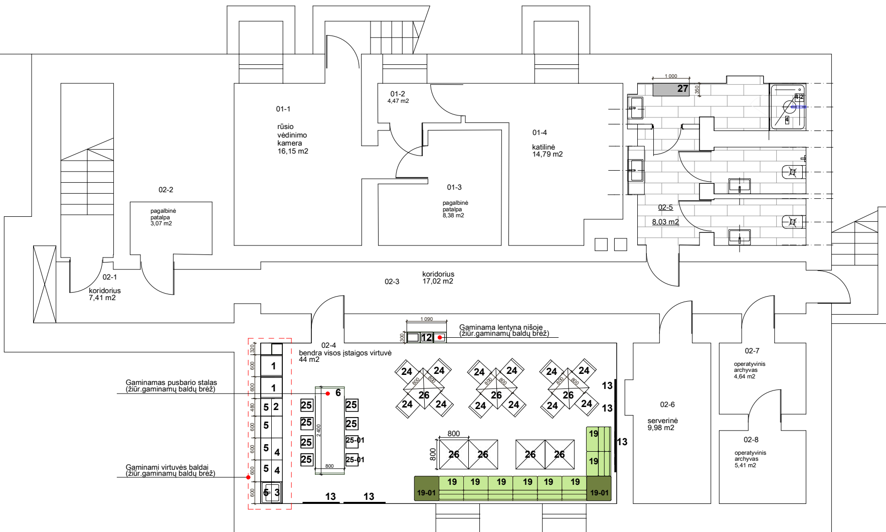
Rūsio planas
