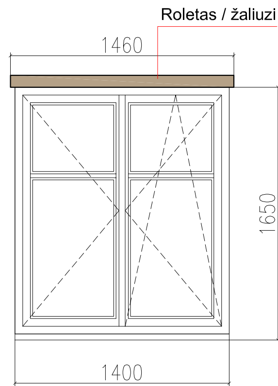
Darbo kabineto langas 19 vnt. L-1
