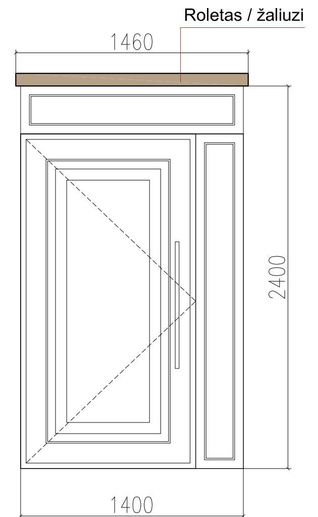
Pasitarimų kambario balkono durys 1 vnt. 2D-1
