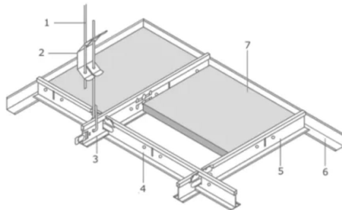
Pakabinamų lubų konstrukcijos elementai:
