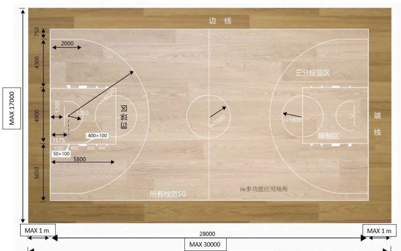
2 pav. Sporto aikštelės matmenys ir linijų ženklavimo pavyzdys
