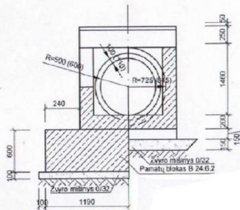
PJŪVIS 2-2, 3-3
