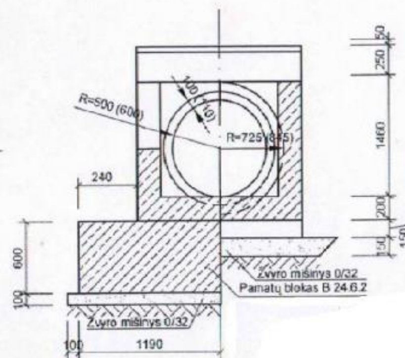
PJŪVIS 2-2, 3-3
