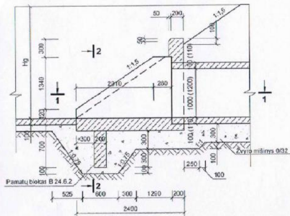
PJŪVIS 1-1
