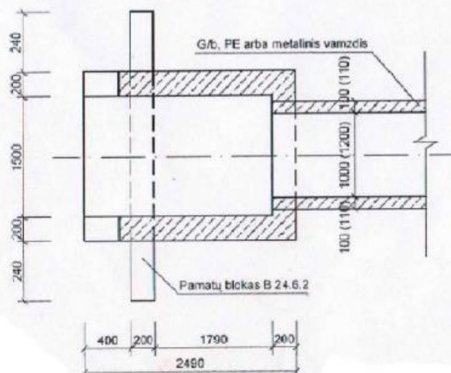
PJŪVIS 1-1
