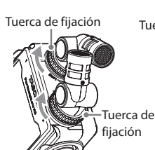
Conexión X-Y
