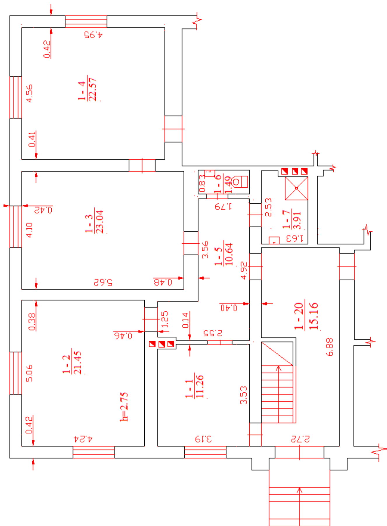
Prezidento g. 7, Tauragė - 2 aukšto planas
