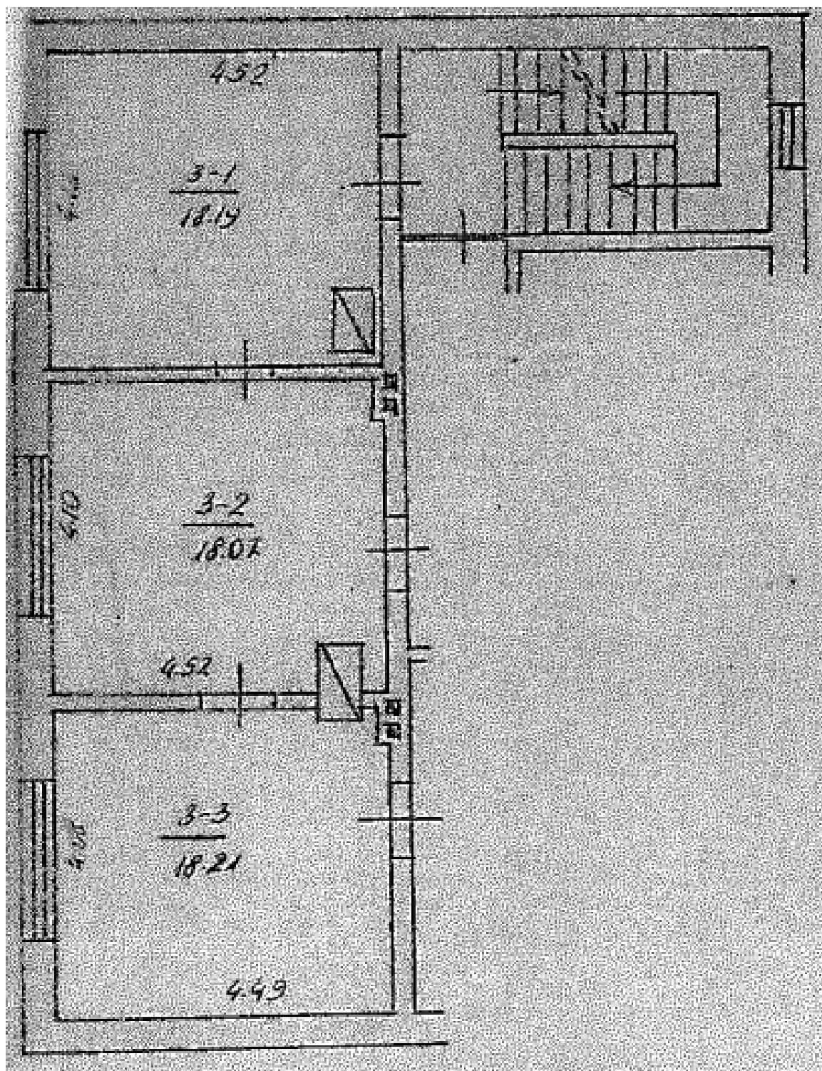
Vilniaus g. 12, Pagėgiai - 2 aukšto plano fragmentas
