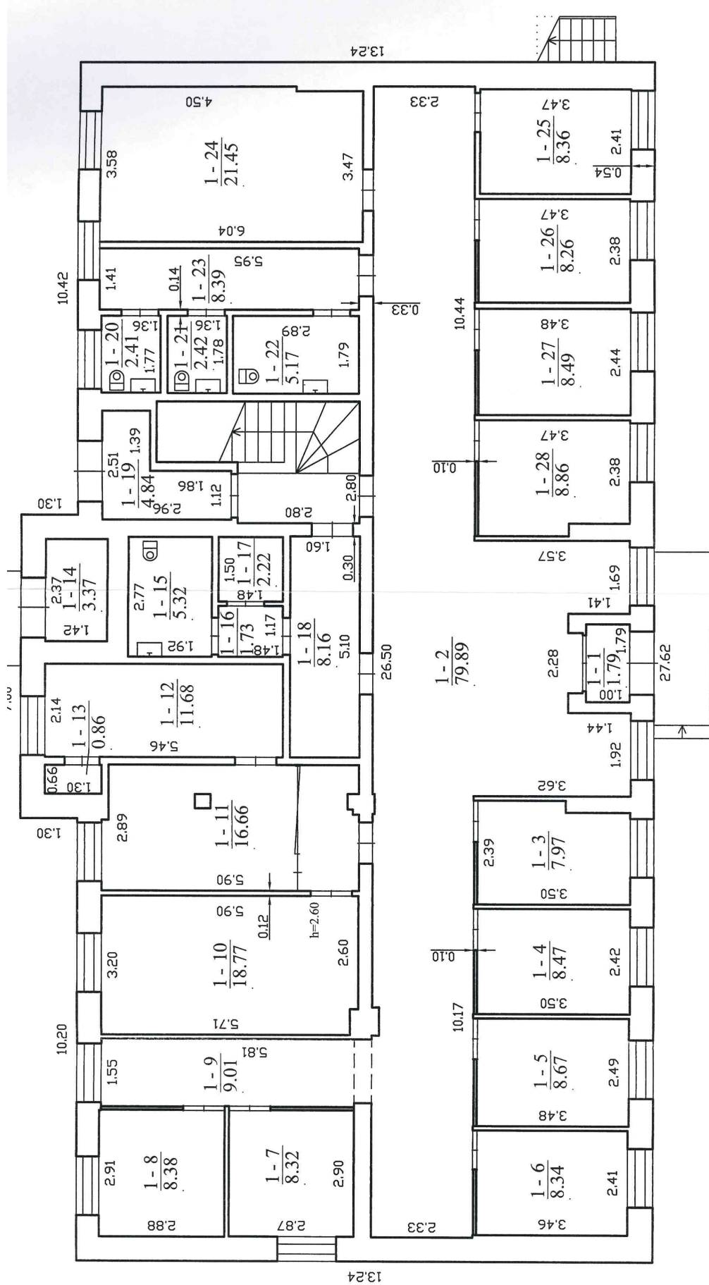
Dariaus ir Girėno g. 54A, Šilalė - 2 aukšto planas
