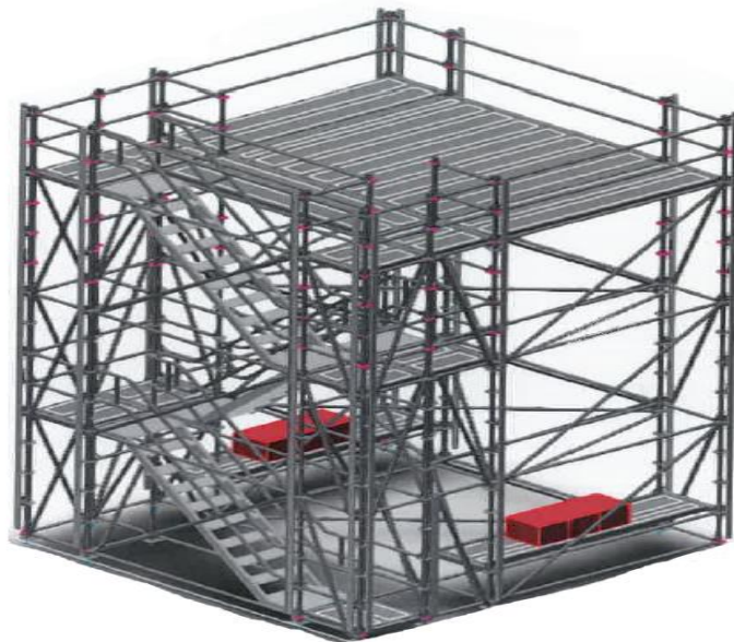
4.3. Pastolių sistemos eskizas
