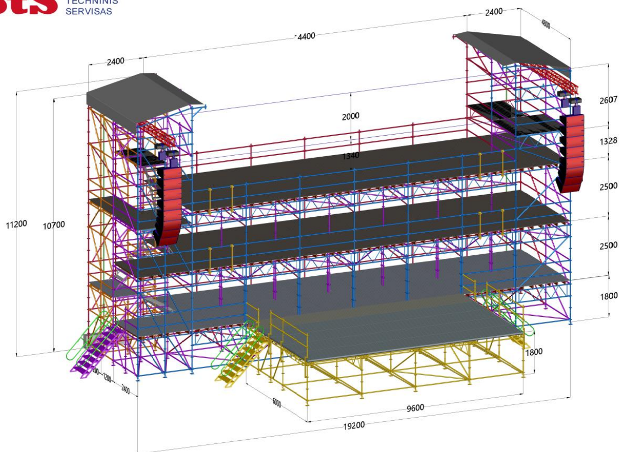
1 pav. Scenos konstrukcija
