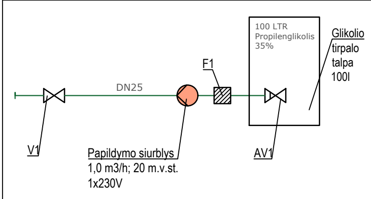
GLIKOLIO PAPILDYMO PRINCIPINĖ PRIJUNGIMO SCHEMA
