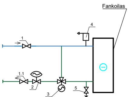
FANKOILS OK-3.01-1; 1.01-4; 1.36; 2.16-2; 2.19-1; 3.21 APRIŠIMO MAZGAS 7/12°C
