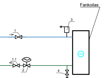
LIKUSIŲ FANKOILŲ APRIŠIMO MAZGAS 7/12°C
