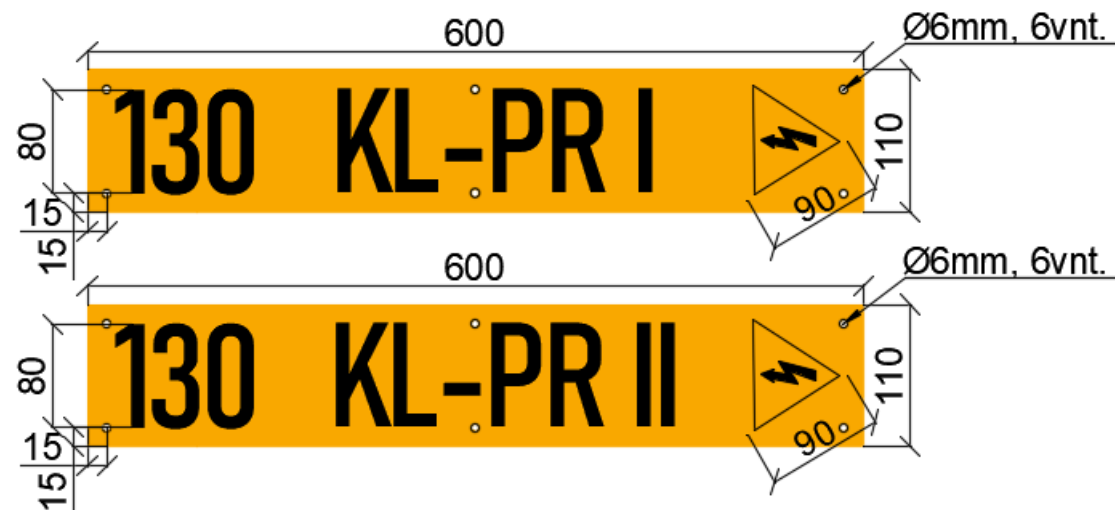
2. 110 kV viengrandės oro linijos atramos žymėjimo lentelė/ Marking plate for pylons of 110 kV voltage one circuit overhead line:
