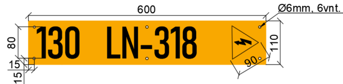
3. 330 kV oro linijos atramos žymėjimo lentelė/ Marking plate for pylons of 330 kV voltage overhead line:
