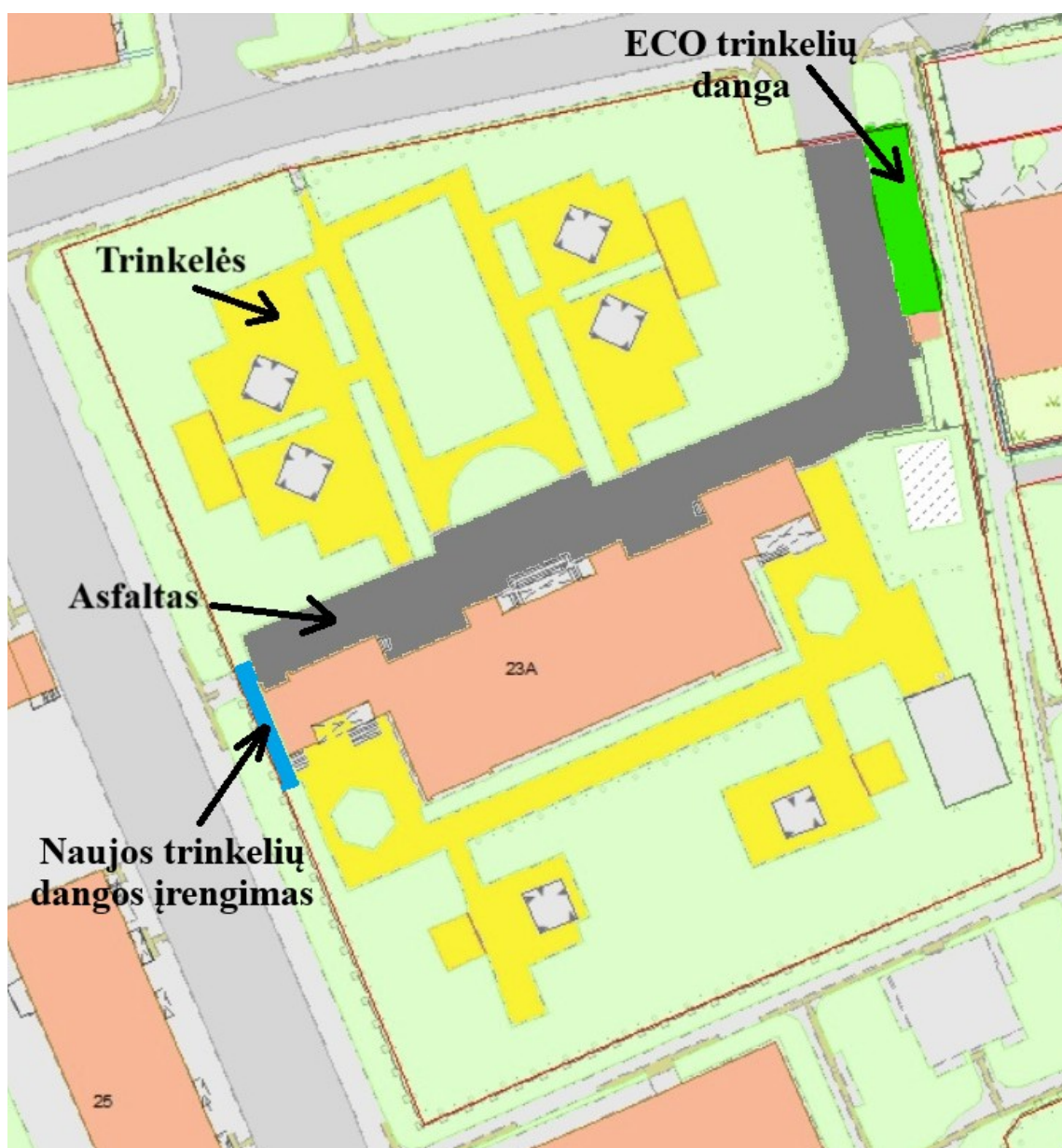
1 pav. Teritorijos remontuojamų dangų schema (geltona spalva – trinkelės danga; pilka spalva –
